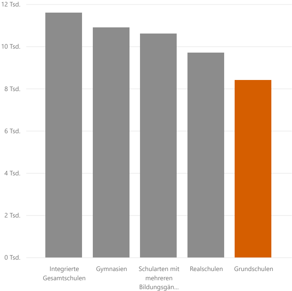
Ausgaben Schulart (DE 2023) nach schulart
