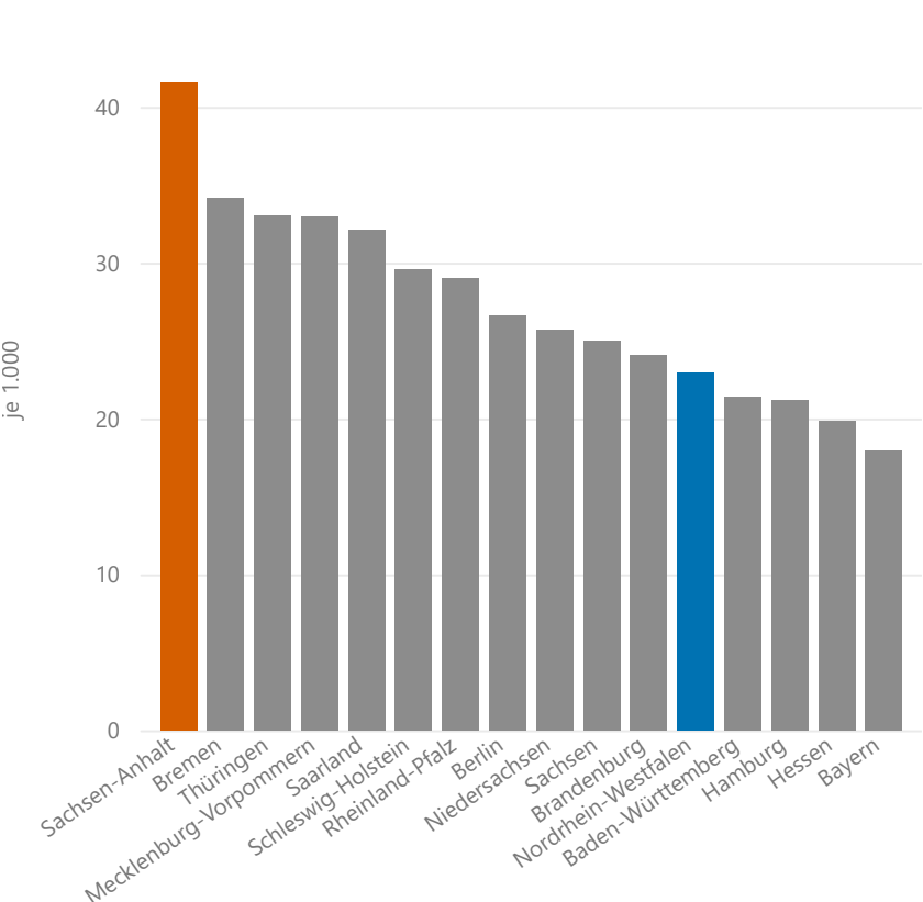
Ohne HSA je 1000 (15-18) nach region
