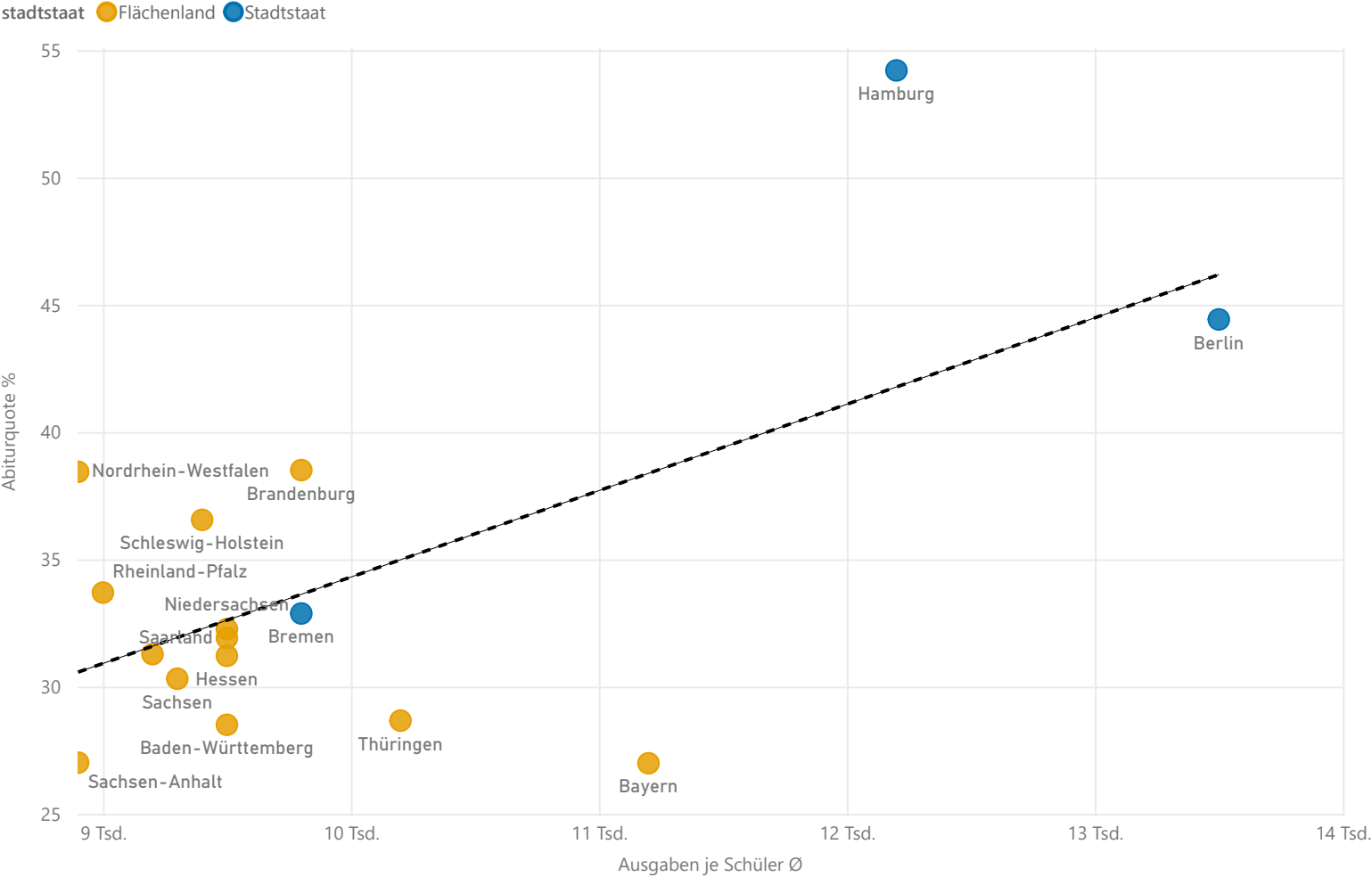
Ausgaben je Schüler Ø und Abiturquote % nach region und stadstaat
