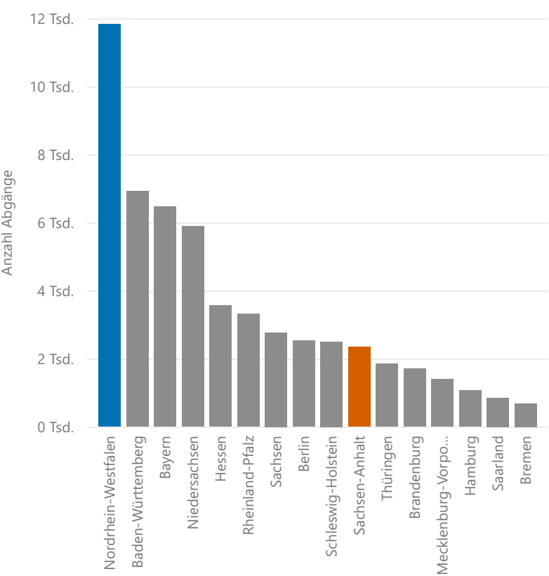
Abgänge ohne HSA nach region
