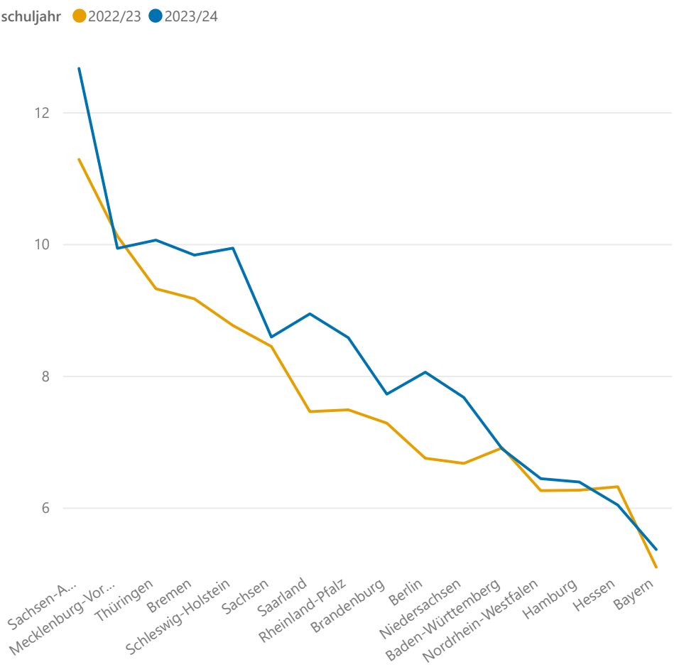
Quote ohne HSA % nach region und schuljahr
