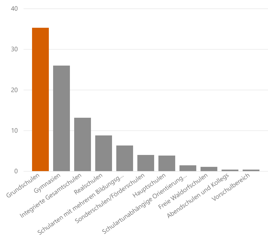
Schüleranteil % nach schulart
