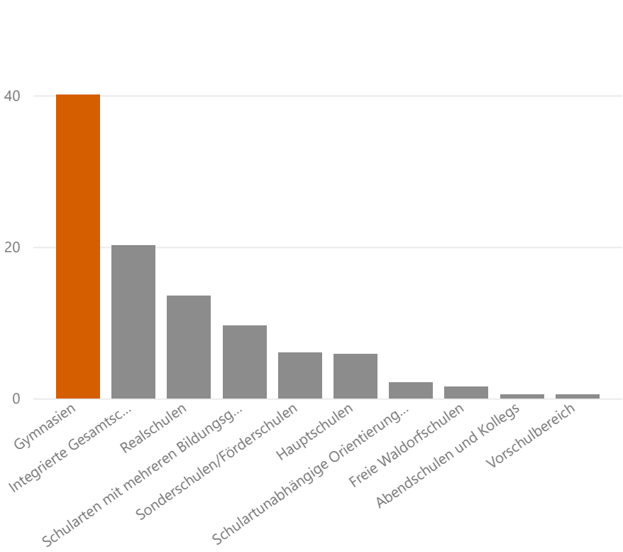
Schüleranteil ohne Grundschule % nach schulart
