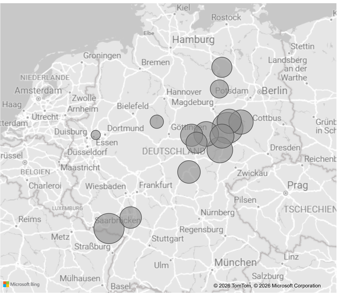
Quote ohne HSA % nach Kreis
