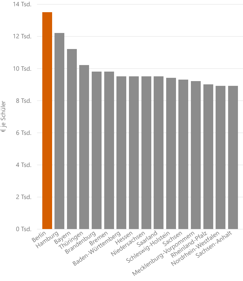
Ausgaben je Schüler (2023) nach Land
