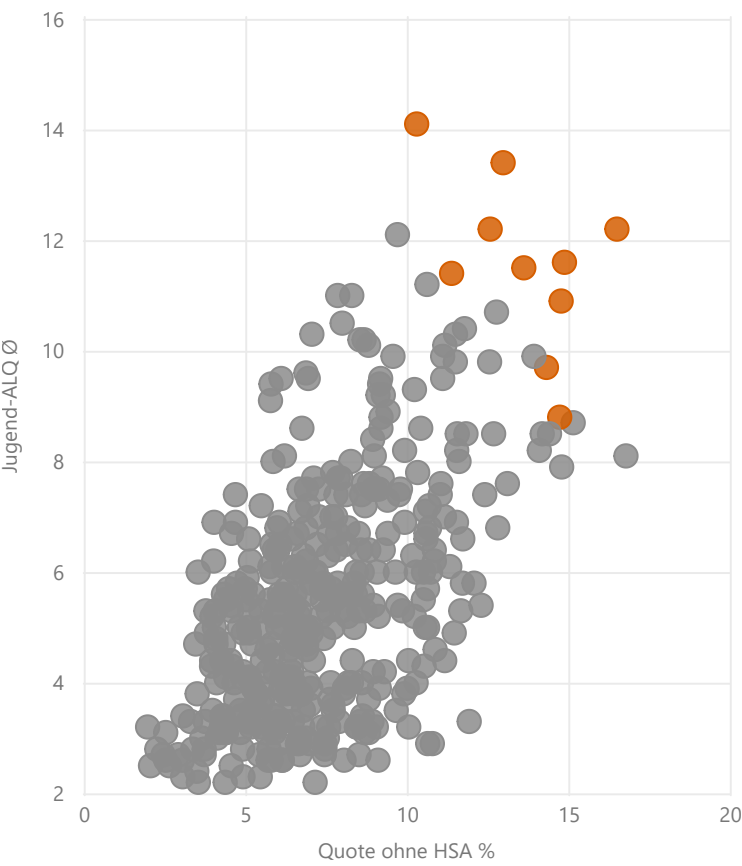
Quote ohne HSA %, Jugend-ALQ Ø, Risiko-Score und Verf. Einkomme...
