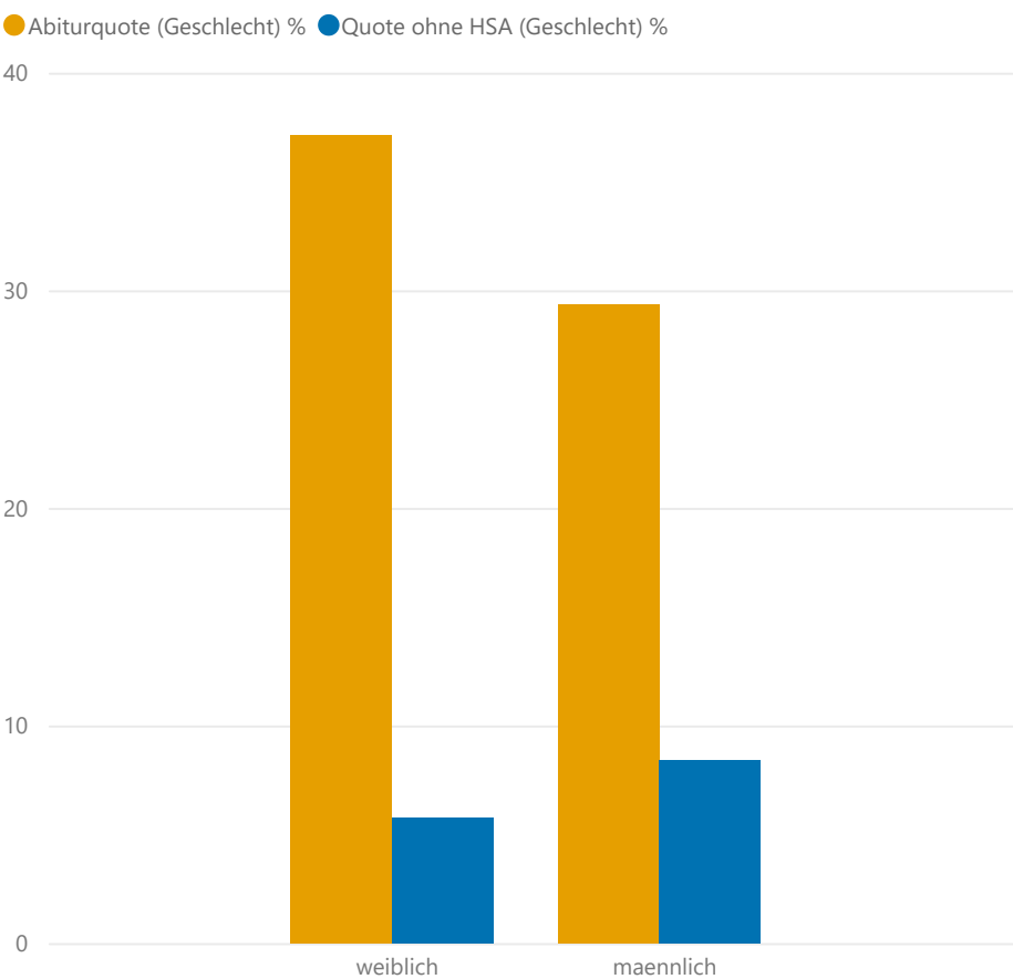
Abiturquote (Geschlecht) % und Quote ohne HSA (Geschlecht) % nach geschlecht
