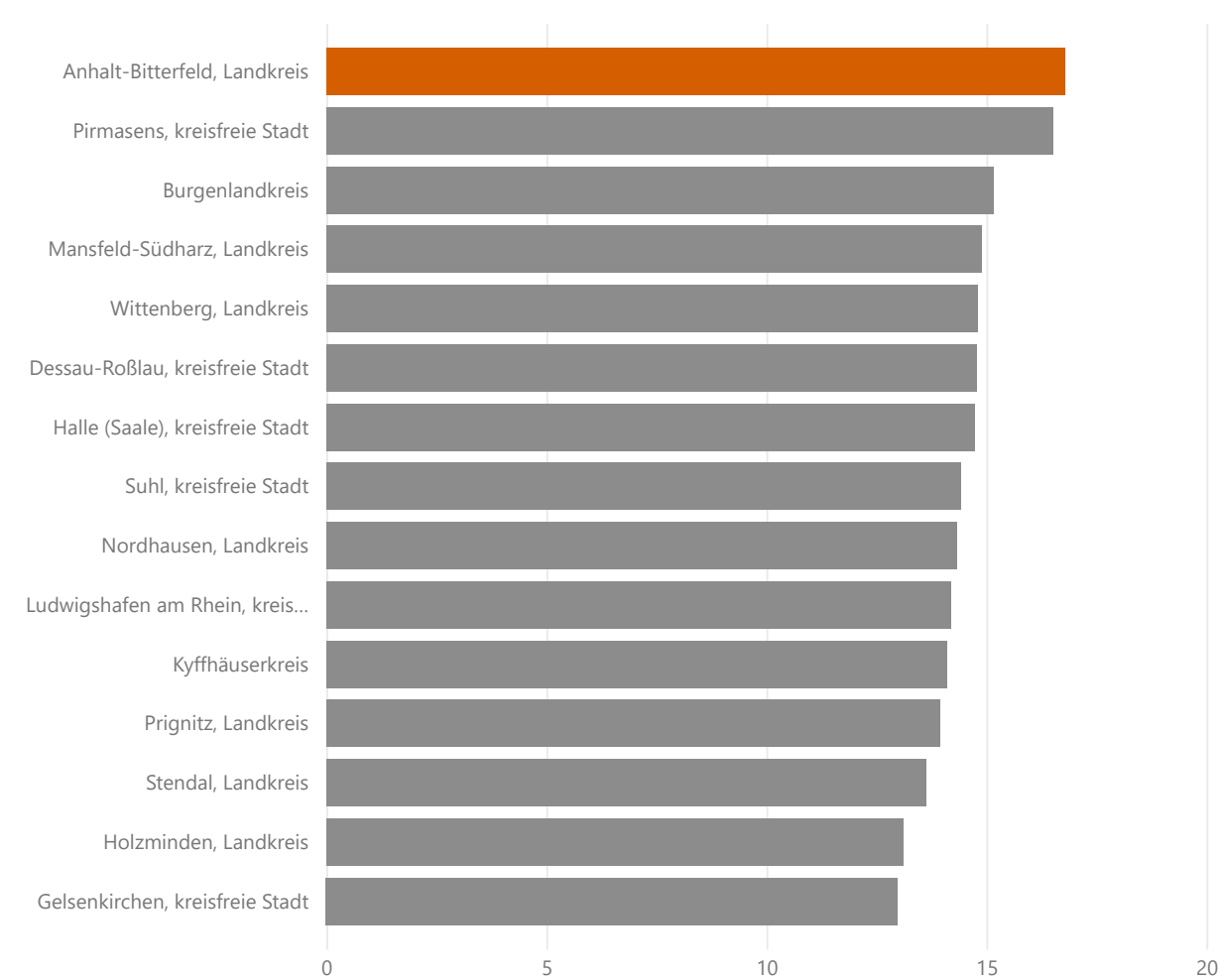
Quote ohne HSA % nach region
