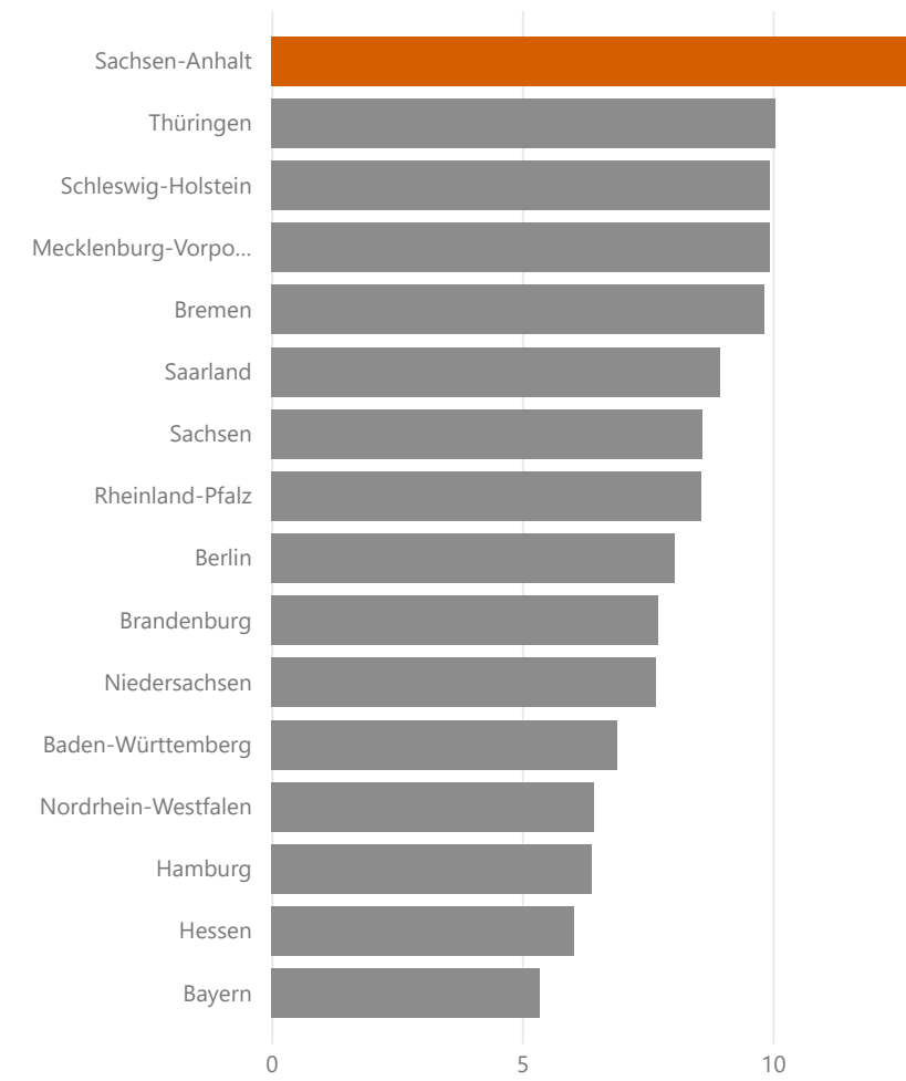
Quote ohne HSA % nach region
