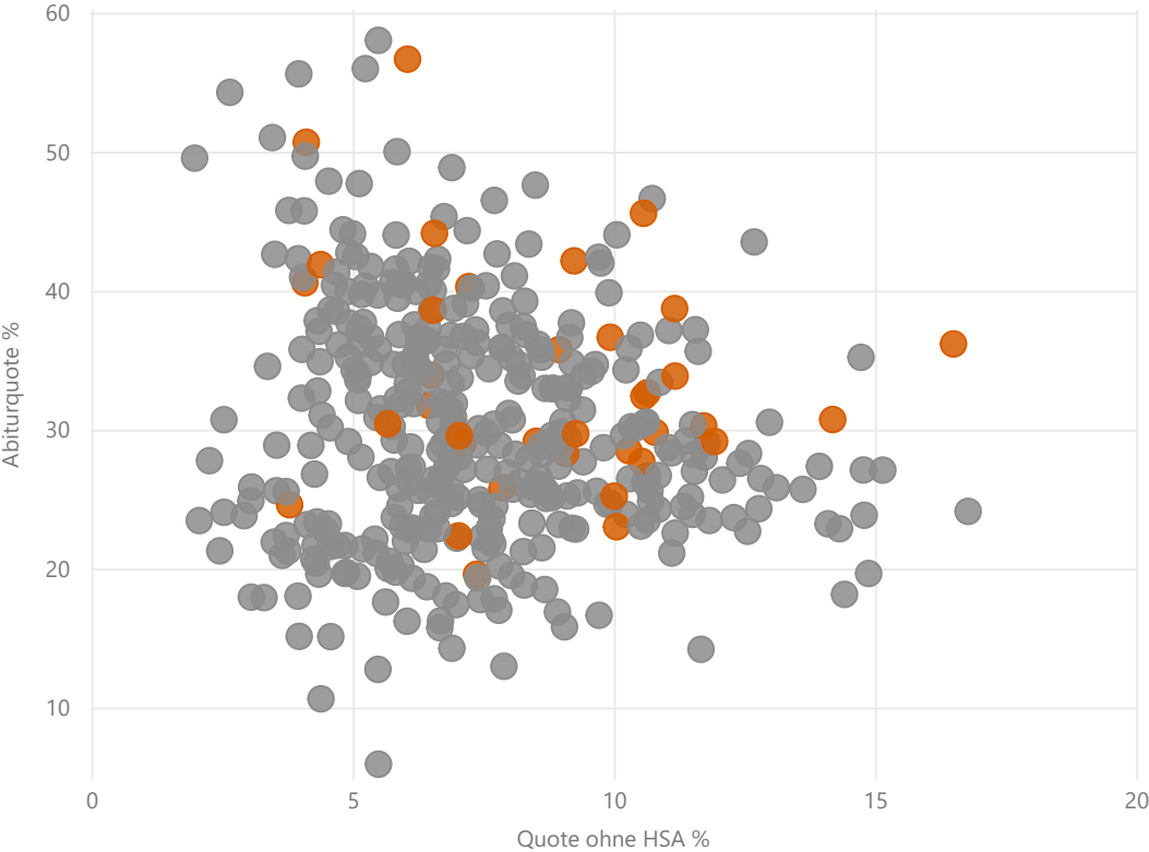
Quote ohne HSA % und Abiturquote % nach region
