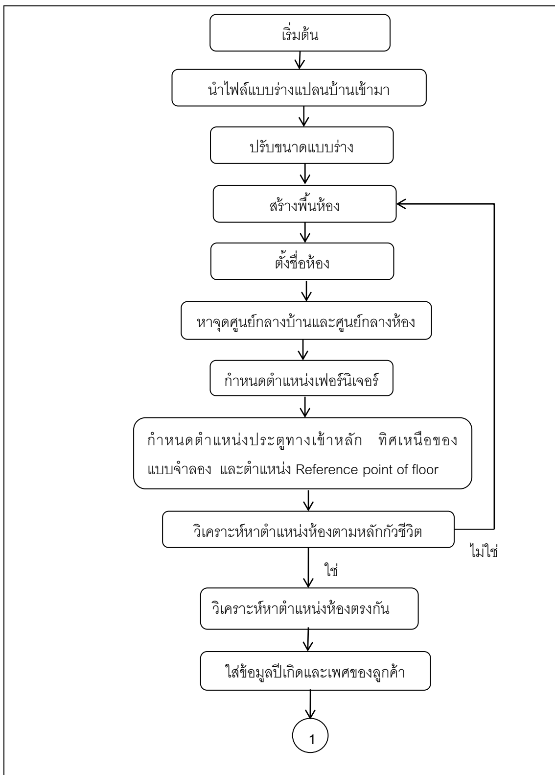
ภาพที่ 66 แผนผังการทำงานของโปรแกรมระบบวิเคราะห์แบบร่างสถาปัตยกรรมภายในตามหลัก
