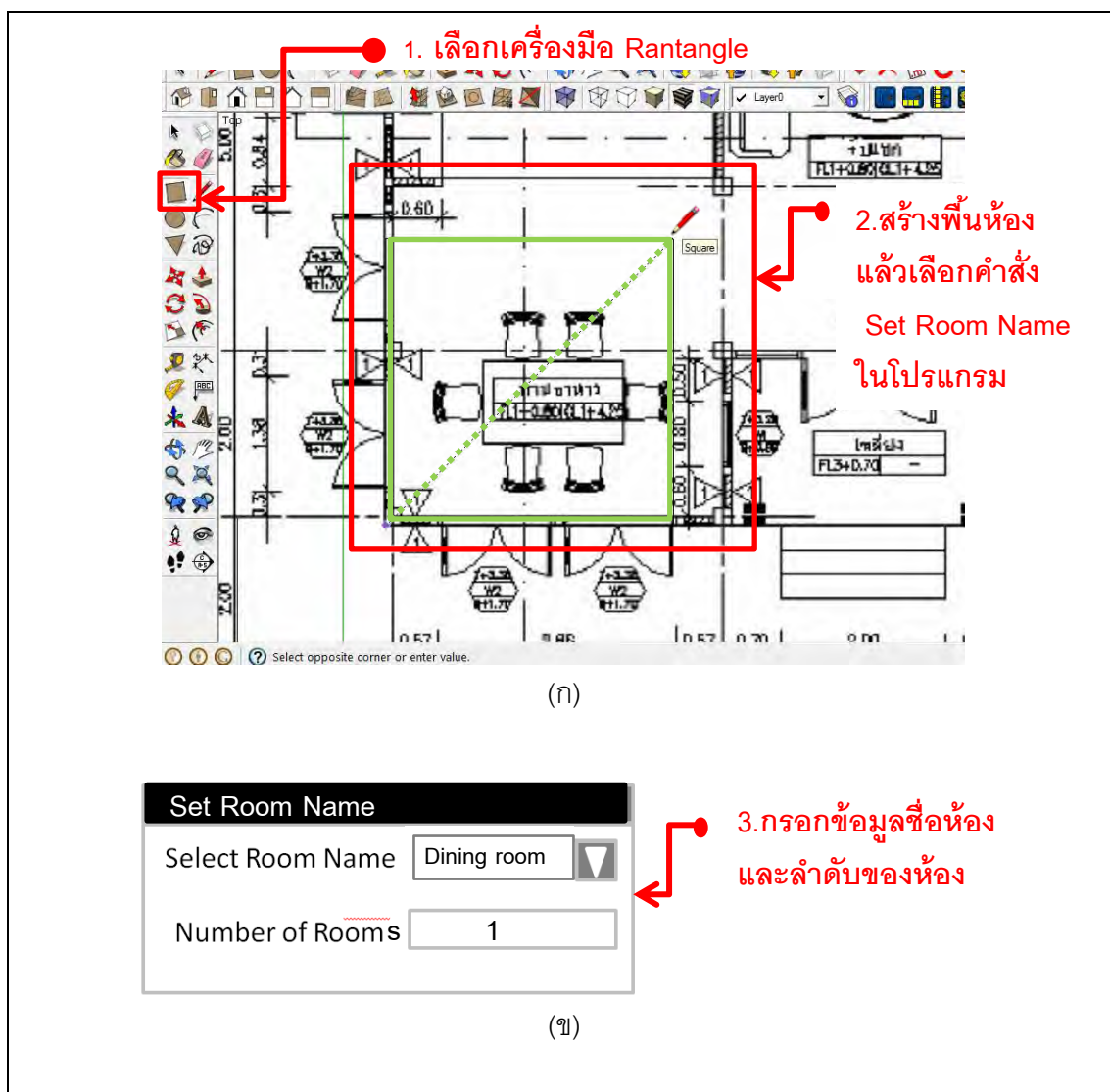
ภาพที่ 72 ตัวอย่างการสร้าง Face ของพื้นห้อง และการกำหนดชื่อห้อง
