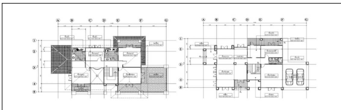
ภาพที่ 18 แสดงแปลนโครงการบ้านพักอาศัย 2 ชั้น ขนาด 400 ตร.ม.
