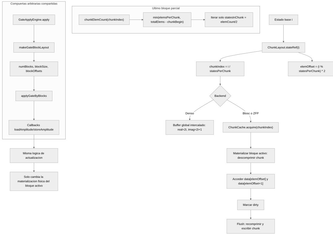
Figura 6: Arquitectura de disposición en bloques y mapeo de estados base en el vector de estado
