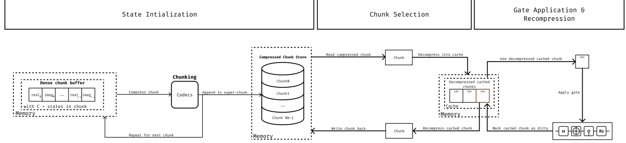
Figura 2: Arquitectura por bloques para la integración de compresión sin pérdida en simuladores cuánticos tipo Schrödinger
