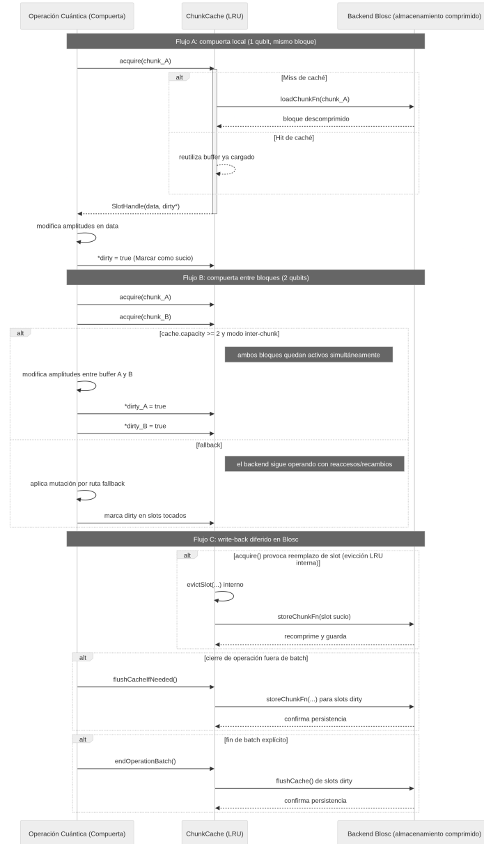
Figura 7: Secuencia operativa del esquema basado en Blosc
