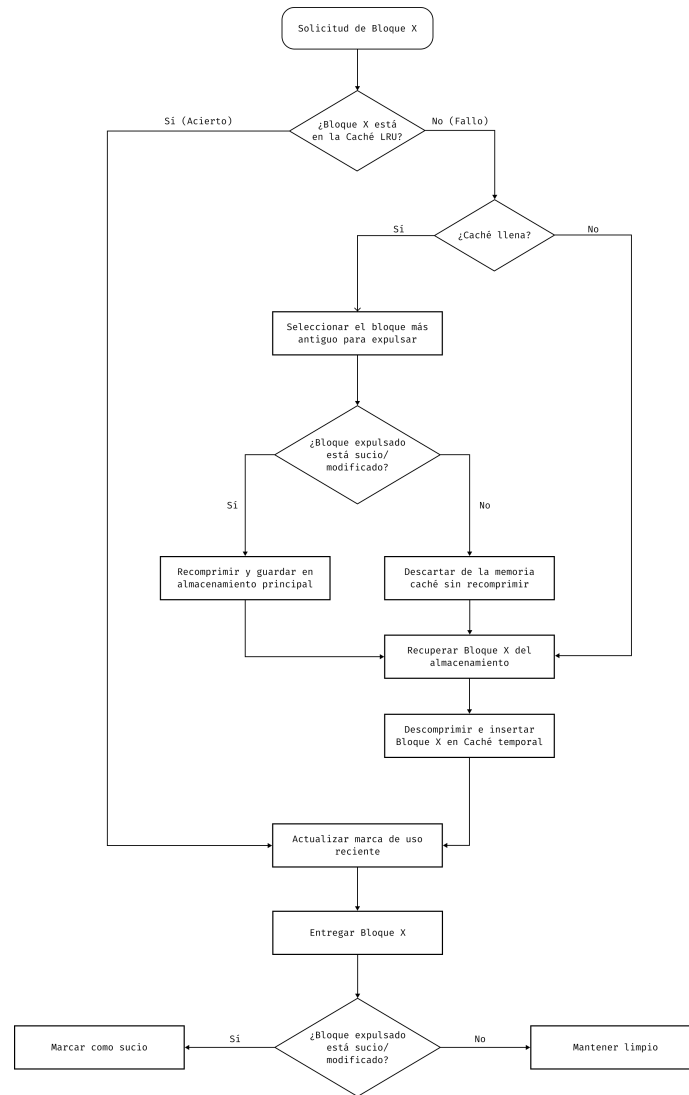
Figura 4: Política de caché LRU para bloques
