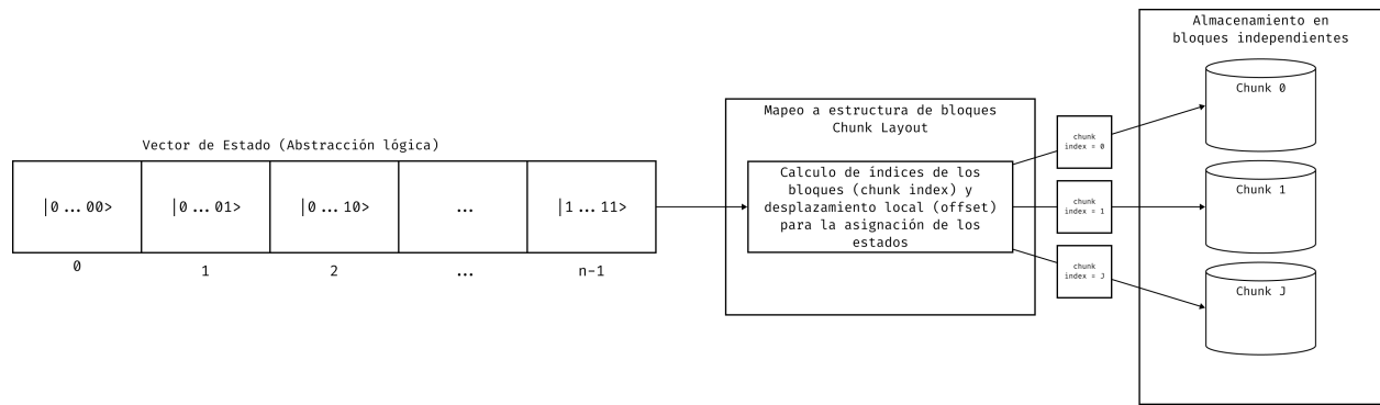
Figura 3: Particionamiento abstracto del vector de estado en bloques independientes
