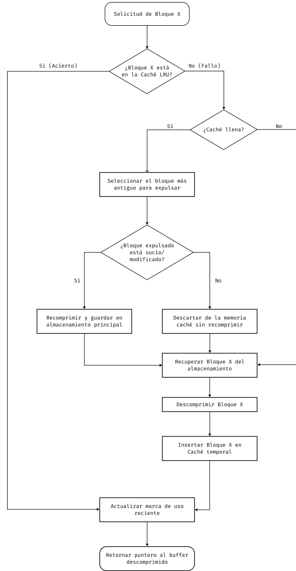
Figura 7: Secuencia operativa del backend basado en Blosc
