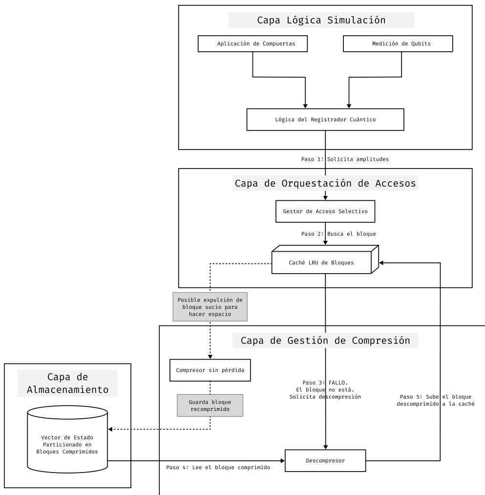
Figura 5: Arquitectura del desarrollo implementado para el backend basado en Blosc
