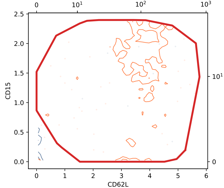
Hierarchy 3
