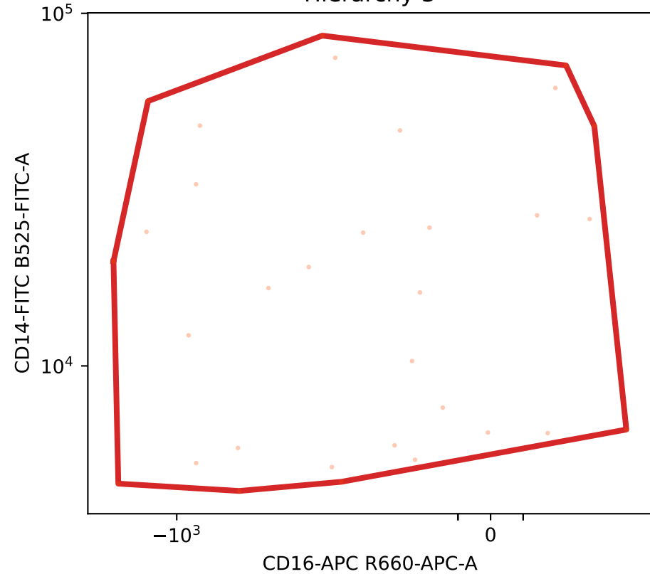
Hierarchy 3
