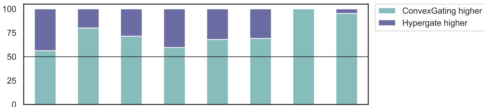
F1
