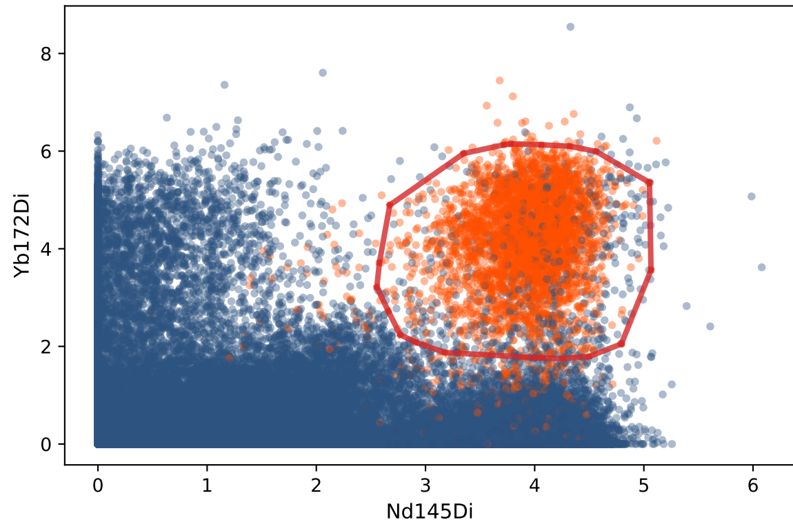
cluster CD4+ TEMRA - hierarchy 1
