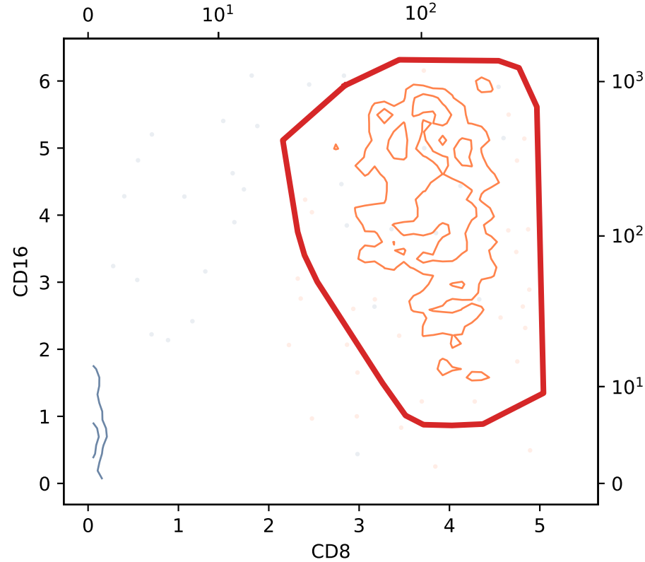
Hierarchy 2
