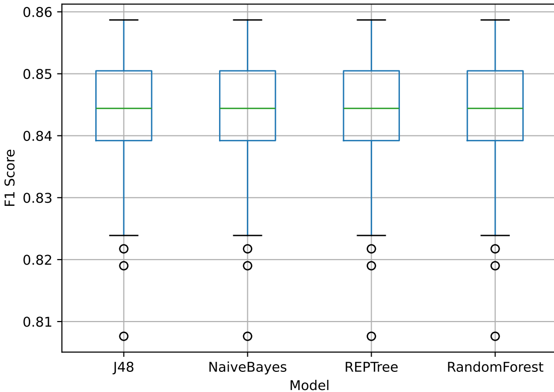
Box and Whisker Plot for F1 Score
