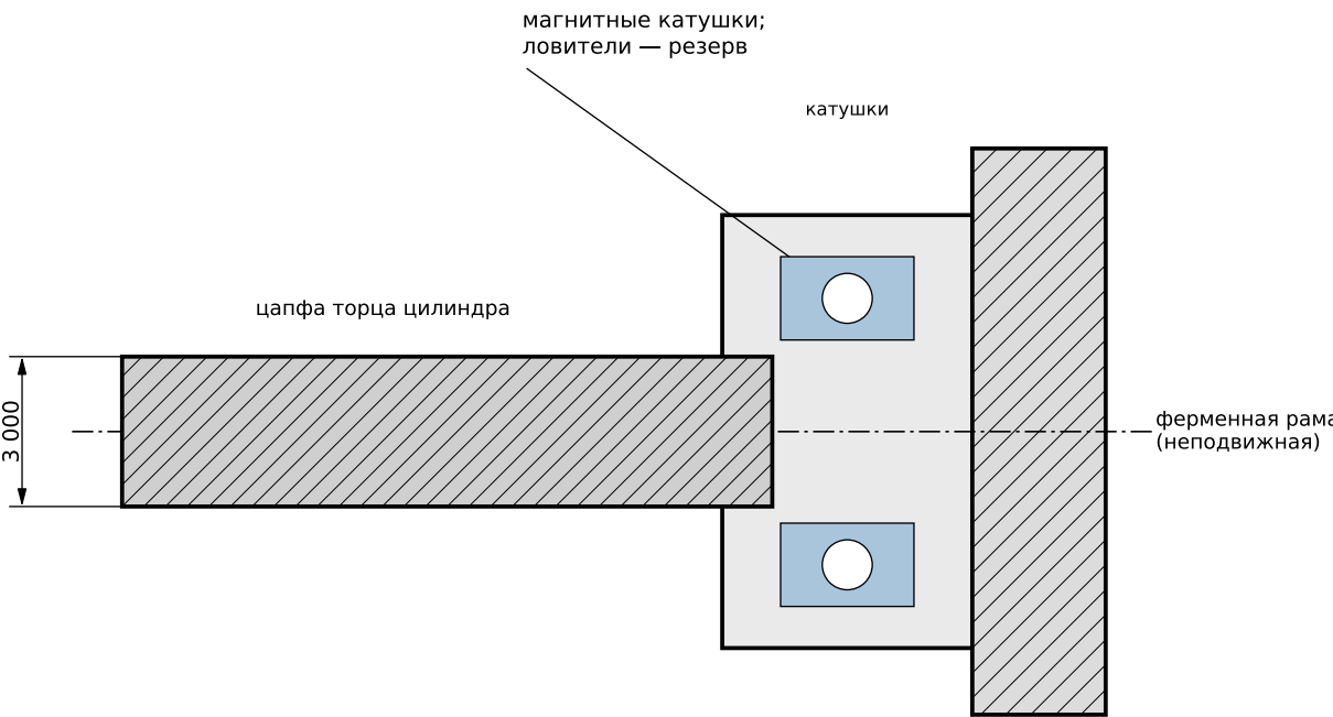
Е (1 : 2 000) подшипниковый узел цапфы
