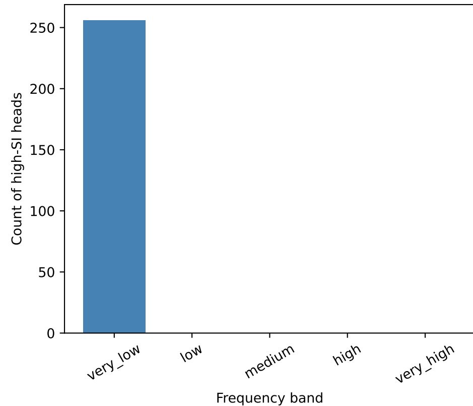
mistral-7b-v0.1
