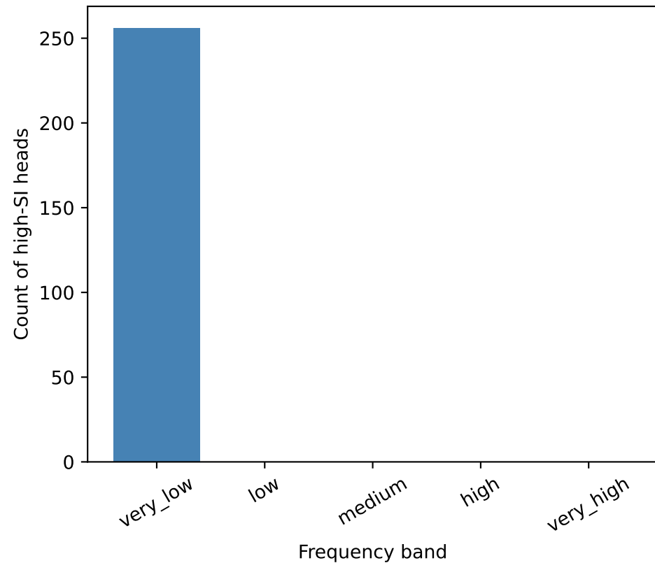
llama-3.1-8b
