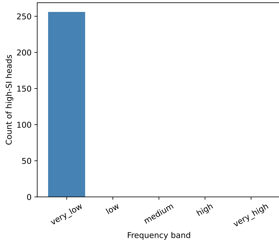
olmo-2-7b
