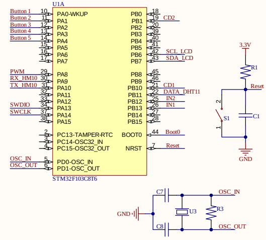
MCU
