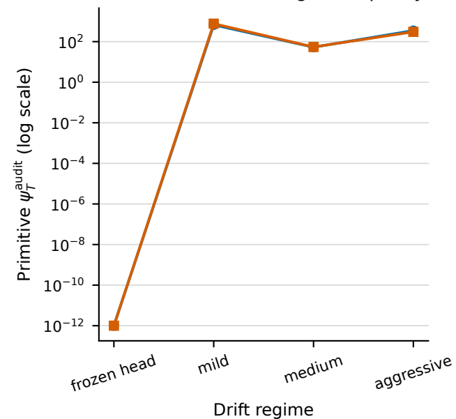
(d) Post-hoc centering discrepancy
