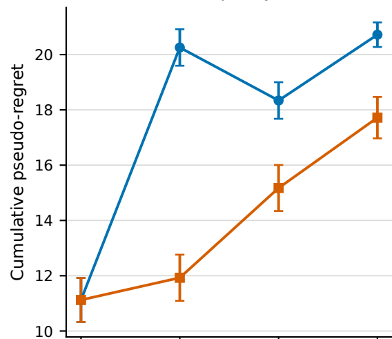
(d) Post-hoc centering discrepancy
