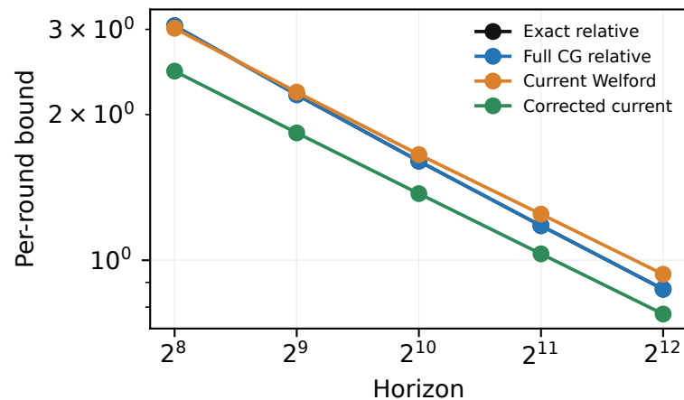
RHS / T
