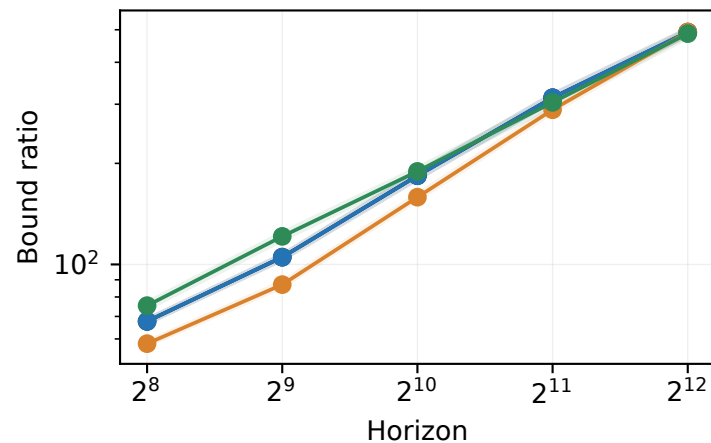
RHS / regret
