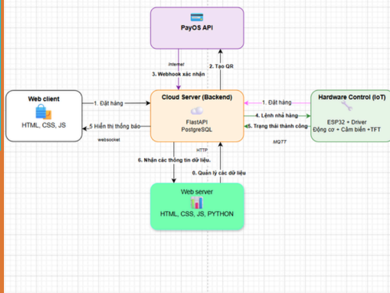
SƠ ĐỒ KIẾN TRÚC HỆ THỐNG
