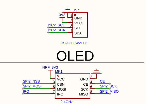
无线通信
