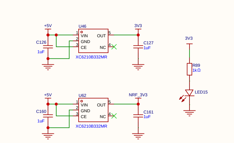
LDO3V3
