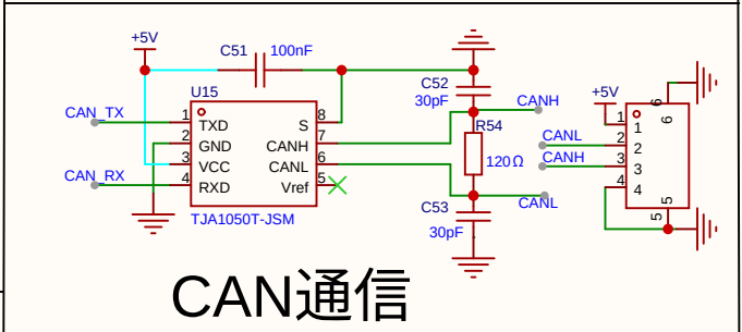
外部通讯
