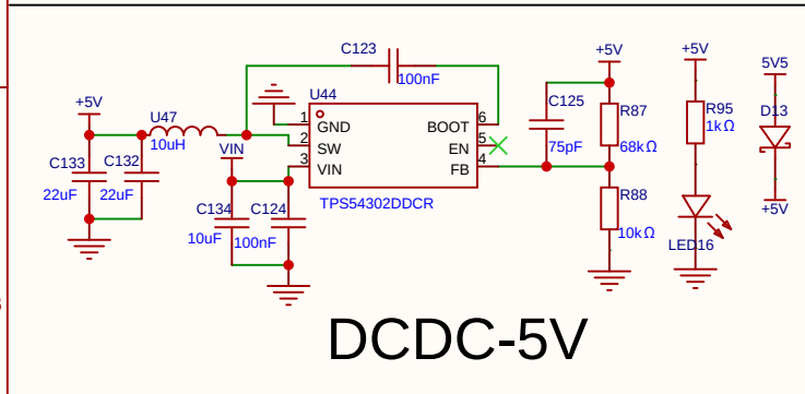
电源输入
