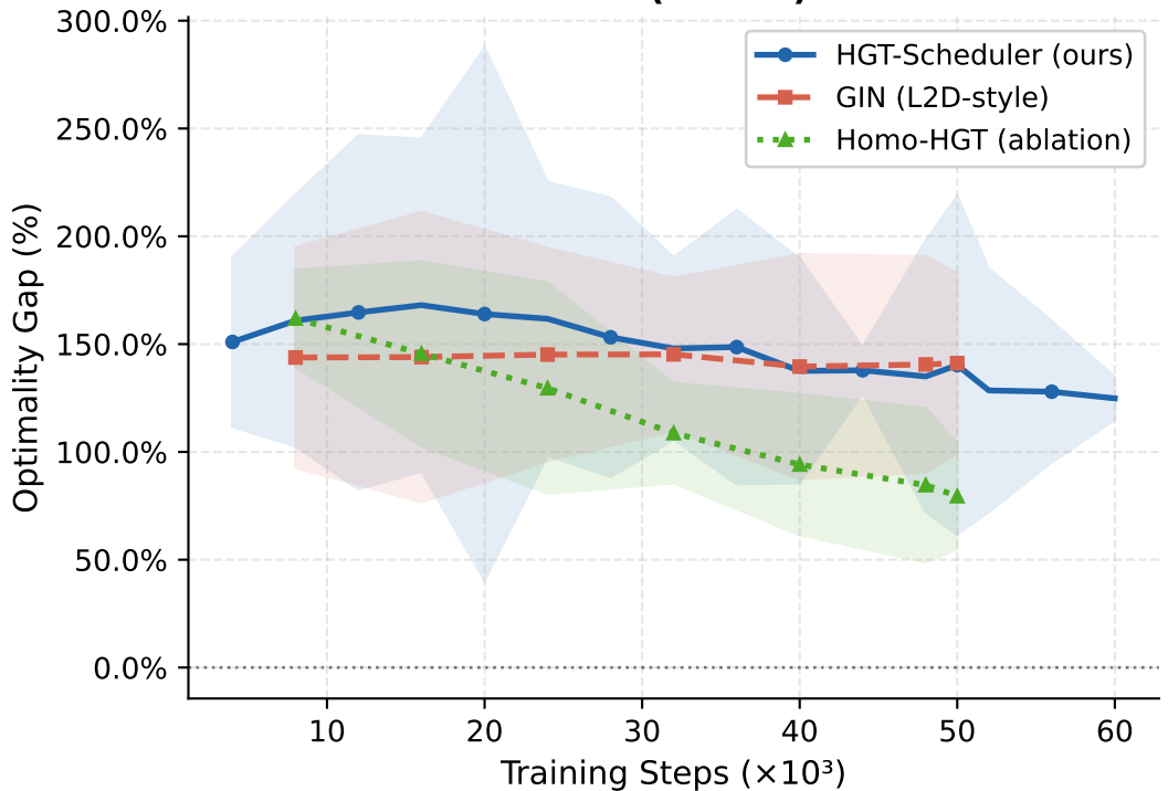
FT10 (10×10)
