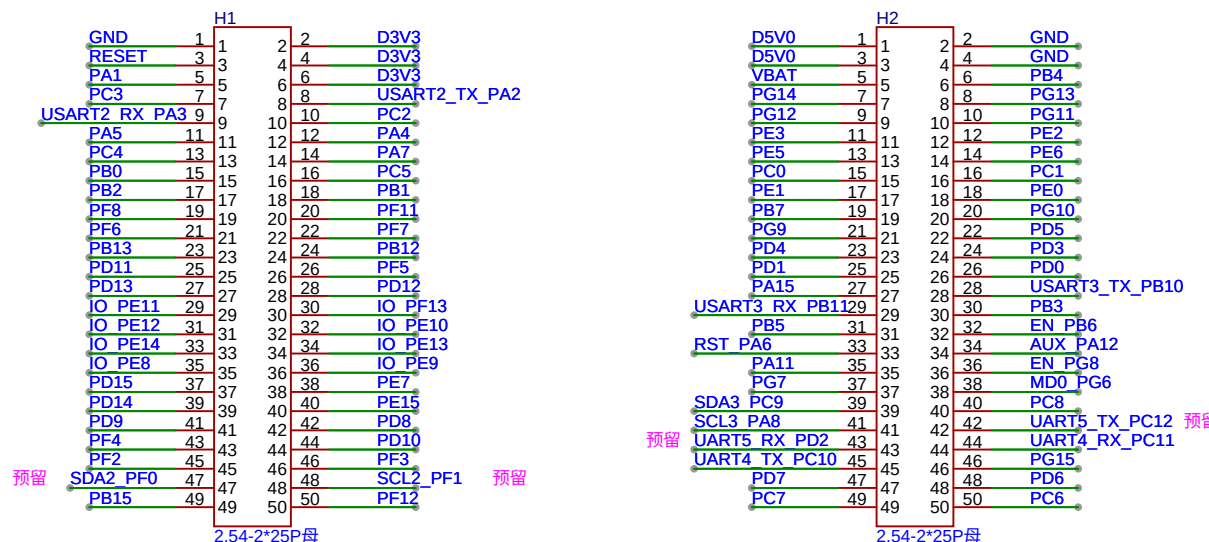
单片机最小系统板接口
