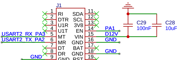
4G模块接口
