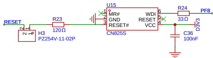
看门狗电路
