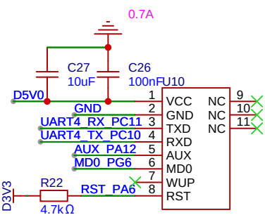
LORA模块接口
