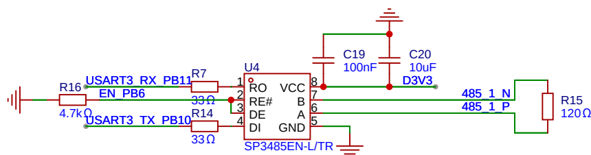
485传感器通信
