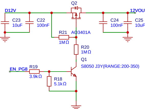
传感器供电开关
