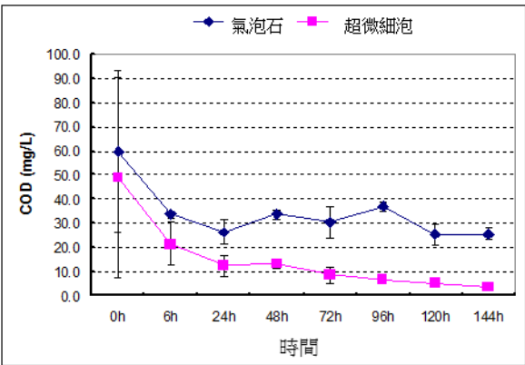
超微細泡對分解 COD 構成有機物的影響
