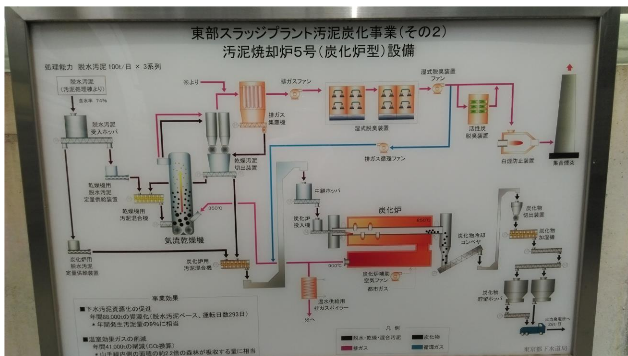
東部污泥處理公司-污泥碳化流程
