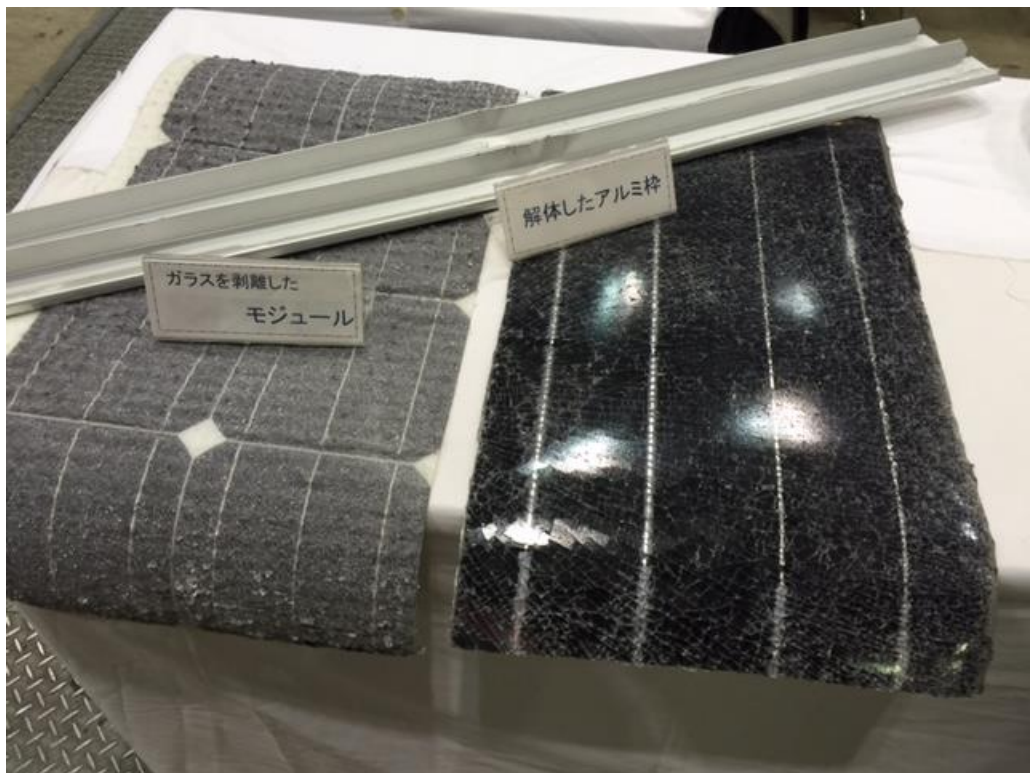
2015 東京環保展-太陽能矽晶板回收
