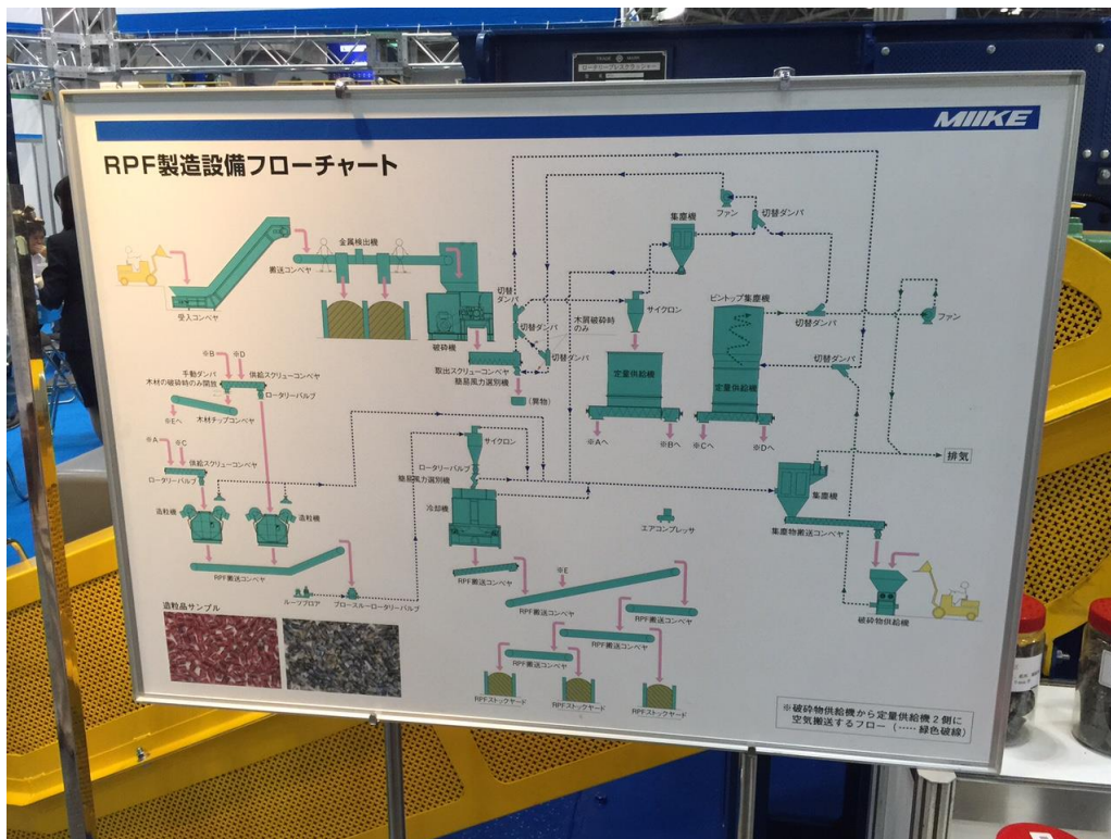
2015 東京環保展-MIKE 公司塑膠固體燃料製造流程
