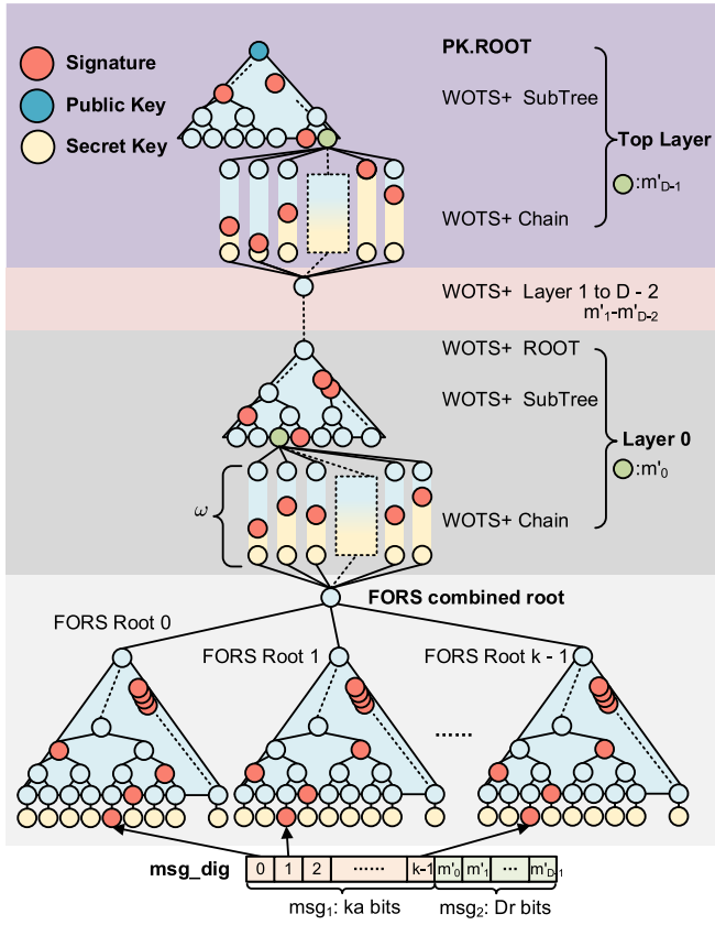
Fig. 2. SPHINCS+ Hypertree.
