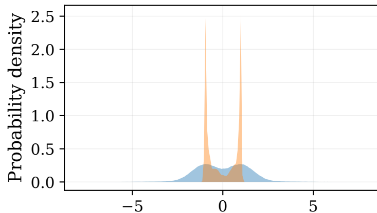
(d) Impulsive
