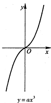
(1) 三次抛物线
