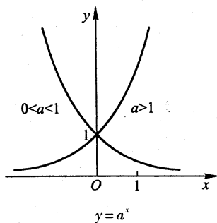
指数函数
