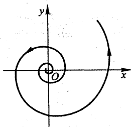
(11) 对数螺线
