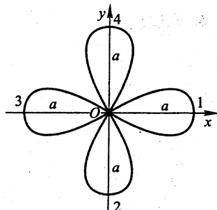
(18) 四叶玫瑰线
