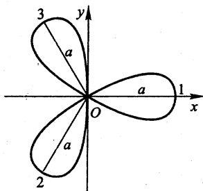
(15) 三叶玫瑰线
