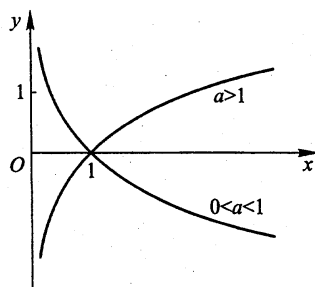
对数函数
