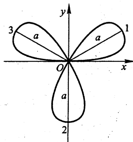
(16) 三叶玫瑰线
