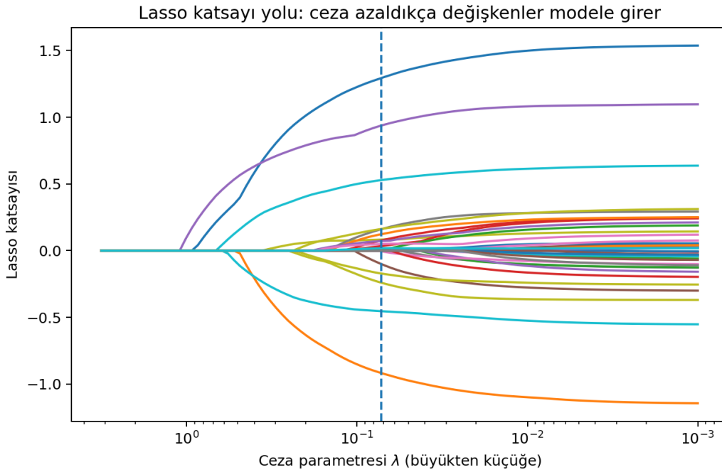
Şekil 11.1: Kontrollü örnekte Lasso katsayı yolu. Kesikli çizgi çapraz doğrulamayla seçilen ceza düzeyini gösterir.
