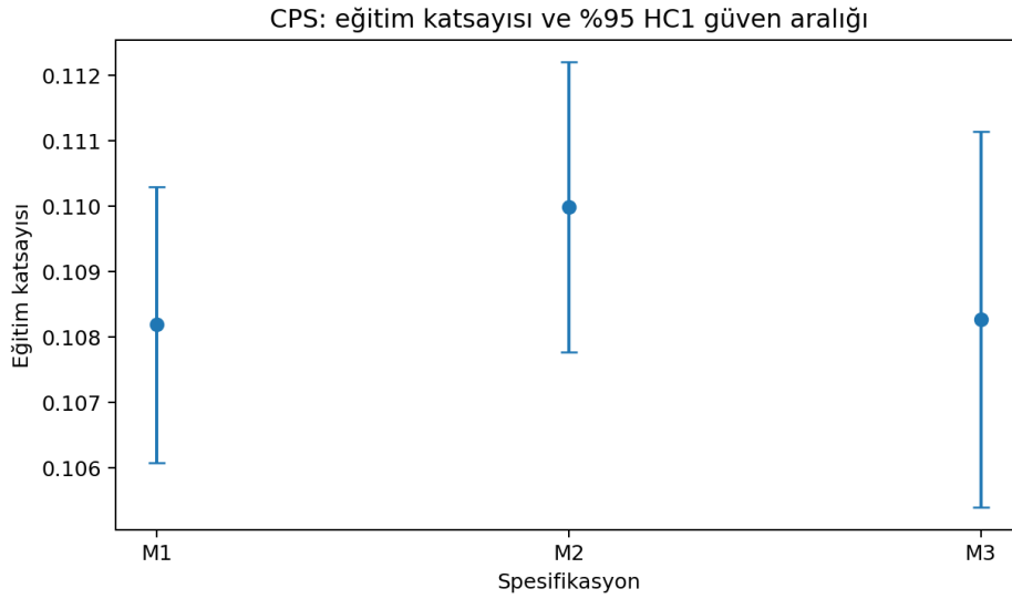
Şekil 2.5: CPS uygulamasında eğitim katsayısının spesifikasyona göre değişimi; çubuklar yüzde 95 HC1 güven aralıklarını gösterir
