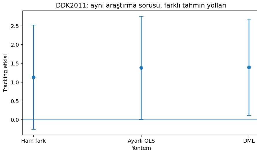
Şekil 12.4: DDK2011: aynı tracking estimand’ı için üç tahmin yaklaşımı
