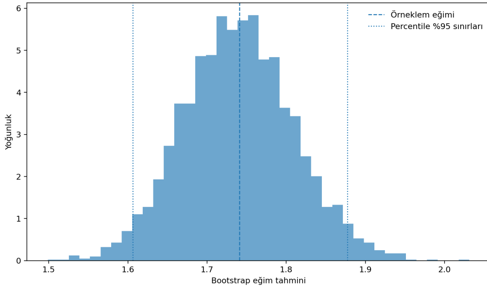
Şekil 10.2: Pairs bootstrap eğim tahminlerinin ampirik dağılımı
