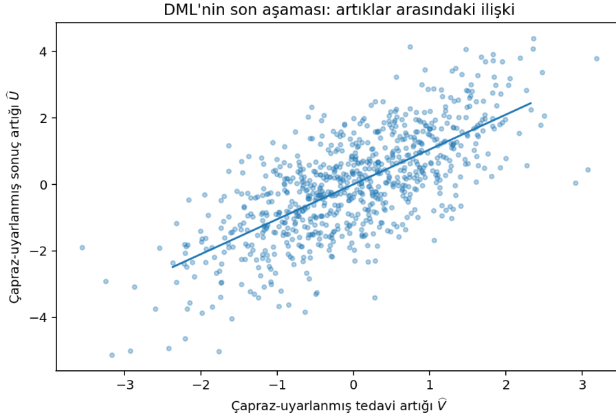
Şekil 12.3: DML son aşamasında çapraz-uyarlanmış sonuç ve tedavi artıklarının ilişkisi. Doğrunun eğimi \hat{\theta}_{DML} 'dir.
