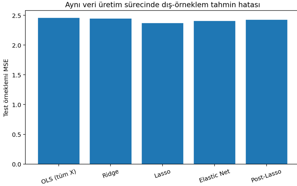
Şekil 11.3: Kontrollü örnekte farklı tahmin edicilerin test örnekleme MSE değerleri.
