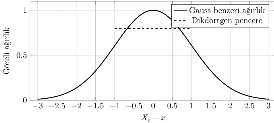
Şekil 8.1: Kernel yaklaşımında merkeze yakın gözlemlerin daha fazla ağırlık alması
