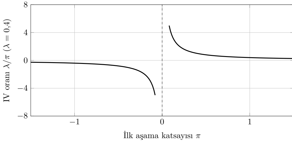
Şekil 4.3: İndirgenmiş biçim etkisi sabitken ilk aşama sıfıra yaklaştığında IV oranının kararsızlaşması
