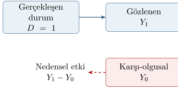
Şekil 3.1: Bir birey için karşı-olgusal sonucun gözlenememesi
