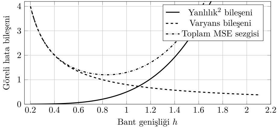
Şekil 8.2: Bant genişliğinde yanlılık–varyans dengesi
