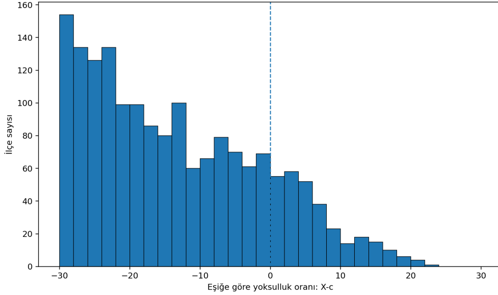
Şekil 9.3: Head Start verisinde eşik değişkeni için eşik çevresi histogramı
