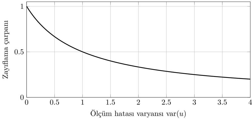
Şekil 3.3: \text{var}(Z) = 1 iken klasik ölçüm hatasının zayıflama çarpanı
