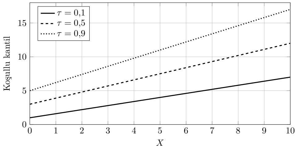
Şekil 7.3: Kantiller boyunca eğim heterojenliği
