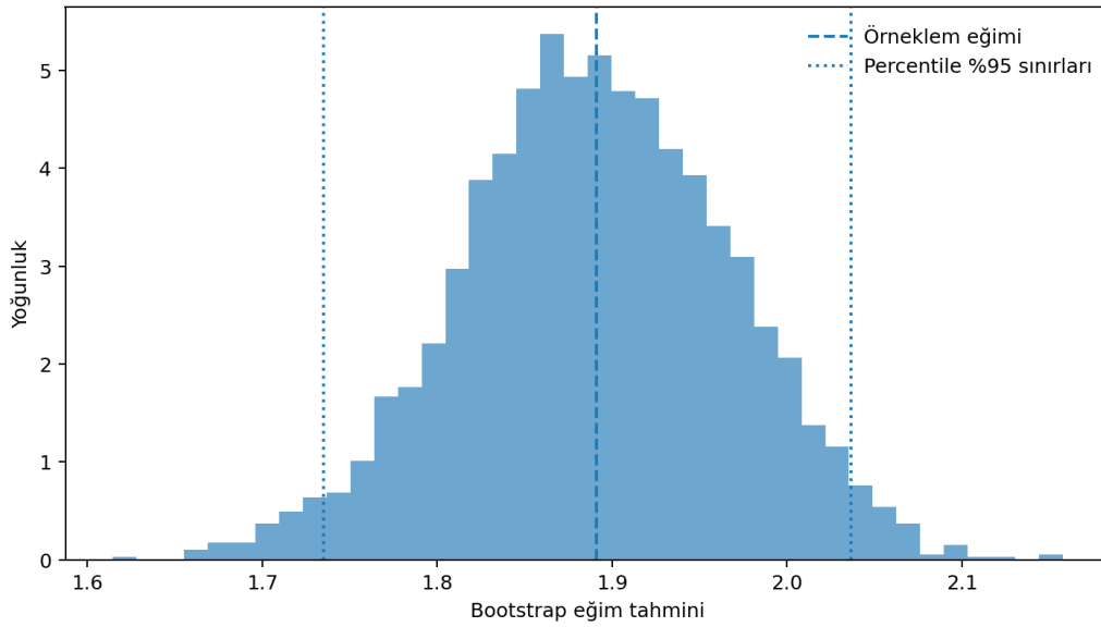
Şekil 10.2: Pairs bootstrap eğim tahminlerinin ampirik dağılımı
