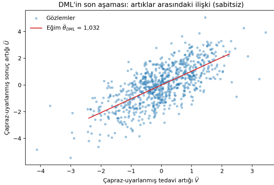
Şekil 12.3: DML son aşamasında çapraz-uyarlanmış sonuç ve tedavi artıklarının ilişkisi. Doğru orijinden geçer; eğimi \hat{\theta}_{DML} 'dir.
