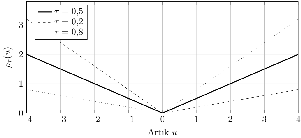
Şekil 7.2: Farklı kantillerde asimetrik check-loss fonksiyonu
