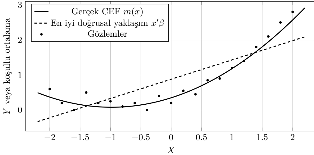
Şekil 1.3: Doğrusal projeksiyon, doğrusal olmayan koşullu ortalamayı yaklaşık olarak özetleyebilir
