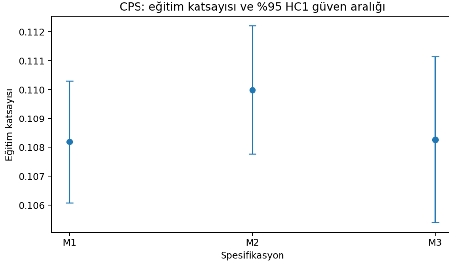
Şekil 2.5: CPS uygulamasında eğitim katsayısının spesifikasyona göre değişimi; çubuklar yüzde 95 HC1 güven aralıklarını gösterir
