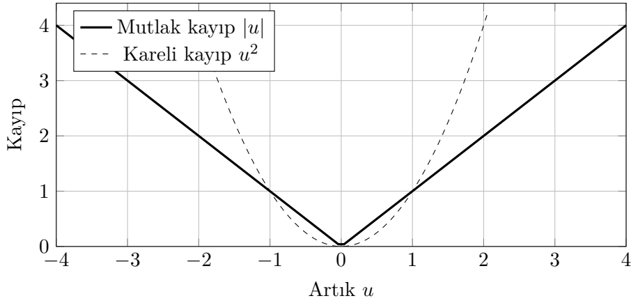
Şekil 7.1: OLS'nin kareli kaybı ile medyan regresyonunun mutlak kaybı
