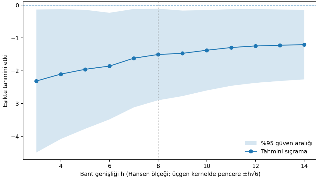
Şekil 9.2: Head Start örneğinde tahmini RDD etkisinin bant genişliğine duyarlılığı
