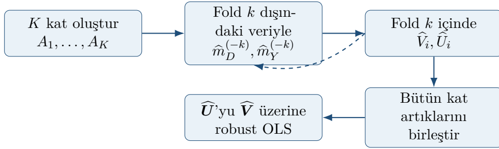
Şekil 12.1: DML çapraz uyarlama (cross-fitting) algoritmasının temel akışı
