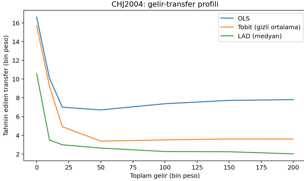
Şekil 6.3: CHJ2004: gelir ve transfer ilişkisinin OLS, Tobit ve LAD ile tahmini
