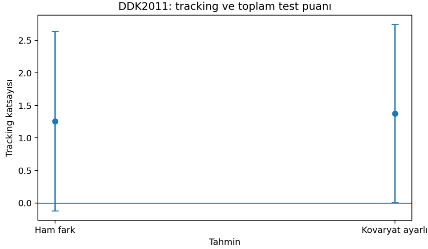
Şekil 3.4: DDK2011 tracking etkisi: ham ve kovaryat ayarlı tahminler
