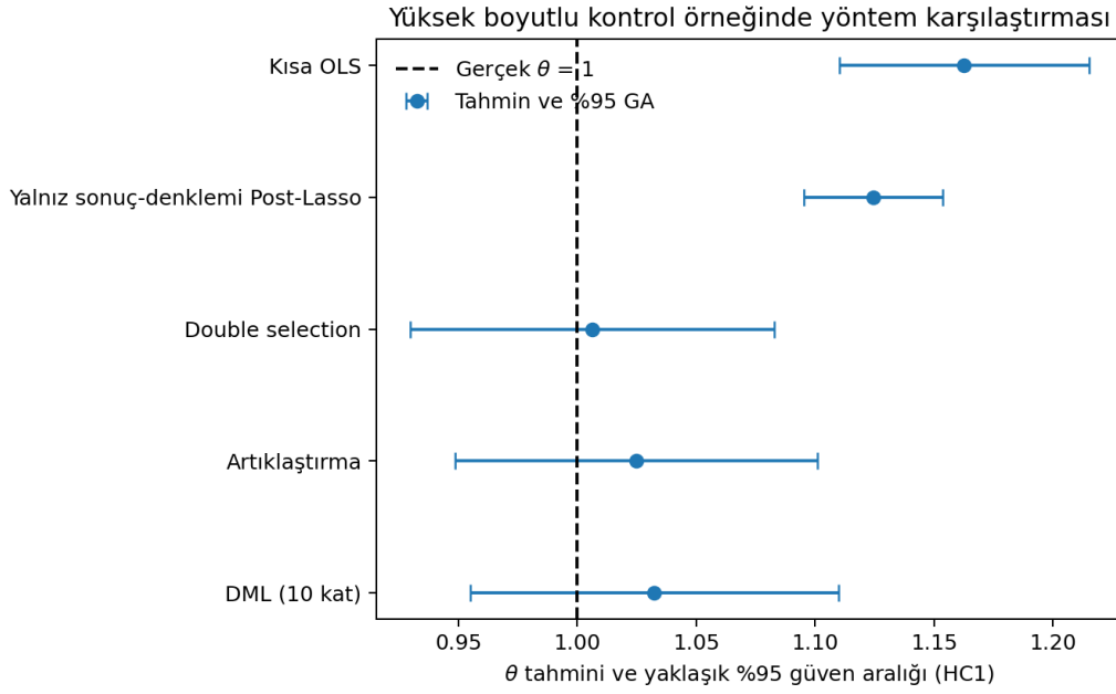
Şekil 12.2: Kontrollü örnekte yöntemlerin \theta = 1 hedefi etrafındaki tahminleri ve yaklaşık yüzde 95 güven aralıkları.
