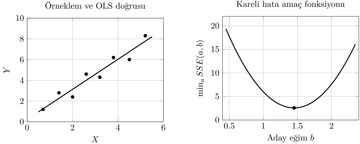
Şekil 1.4: OLS, kareli artıklar toplamını en küçükleyen katsayıyı seçer
