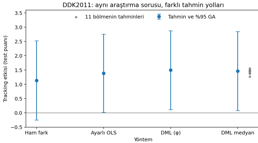
Şekil 12.4: DDK2011: aynı tracking estimand’ı için üç tahmin yaklaşımı. Gri noktalar 11 farklı kat kuralıyla elde edilen DML tahminleridir.
