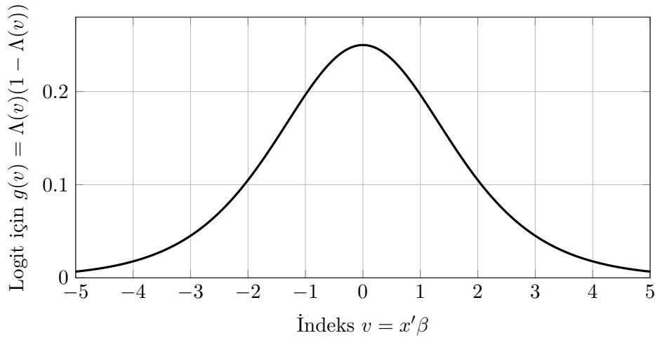
Şekil 5.2: Logit modelinde marjinal etkinin indeks düzeyine göre değişmesi
