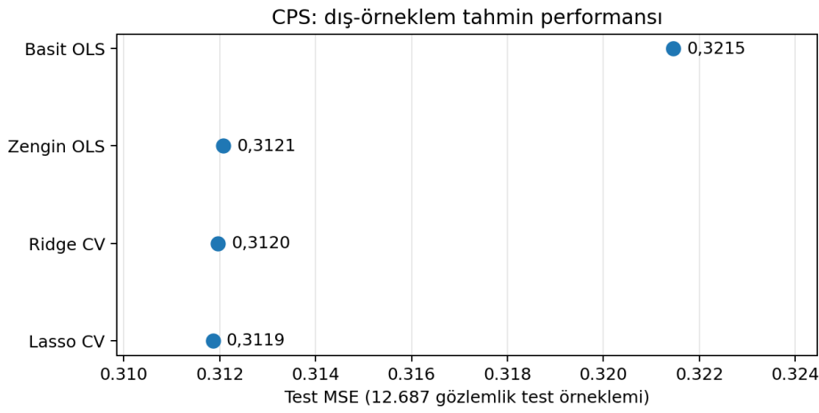
Şekil 11.4: CPS uygulamasında dış-örneklem test MSE karşılaştırması
