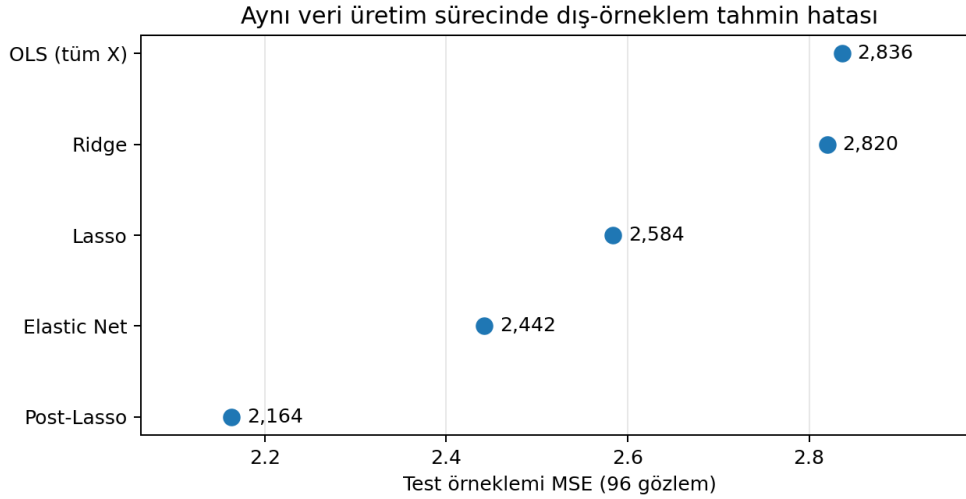
Şekil 11.3: Kontrollü örnekte farklı tahmin edicilerin test örnekleme MSE değerleri.
