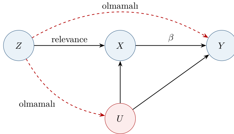
Şekil 4.1: Geçerli aracın temel nedensel yapısı
