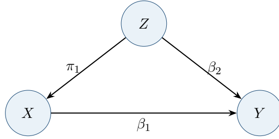
Şekil 2.3: Eksik Z değişkeninin X katsayısını bozabileceği temel yapı
