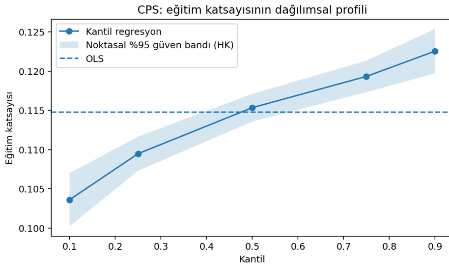
Şekil 7.6: CPS uygulamasında eğitim katsayısının kantil profili ve noktasal yüzde 95 güven bantları
