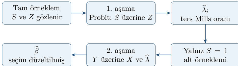
Şekil 6.2: Heckman iki aşamalı seçim düzeltmesinin akışı
