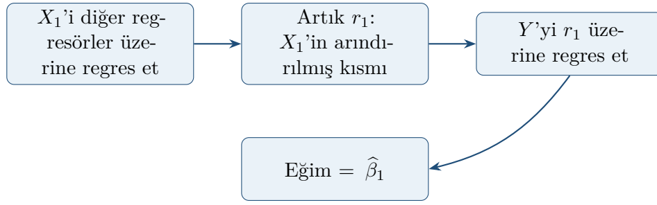
Şekil 2.1: FWL teoreminin kısmi ilişki sezgisi
