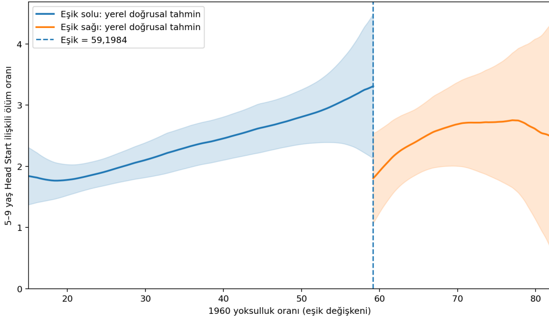
Şekil 9.1: LM2007 Head Start verisinde yerel doğrusal koşullu ortalama tahminleri ve yüzde 95 güven bantları
