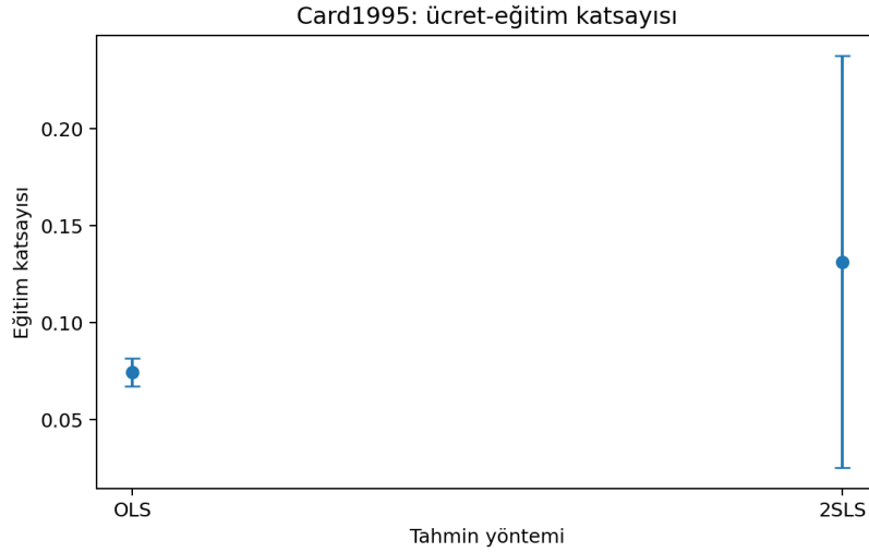
Şekil 4.4: Card1995 uygulamasında OLS ve 2SLS eğitim katsayıları
