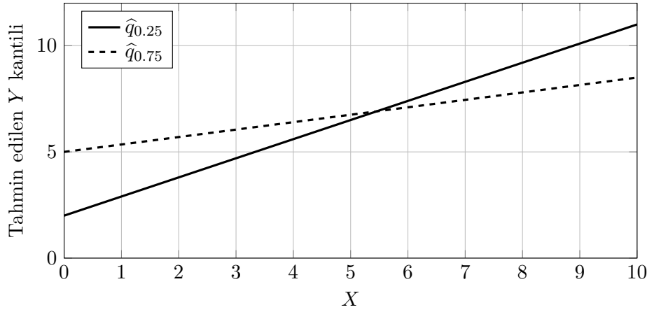
Şekil 7.5: Ayrı doğrusal tahminlerin destek bölgesinde kesişebilmesi
