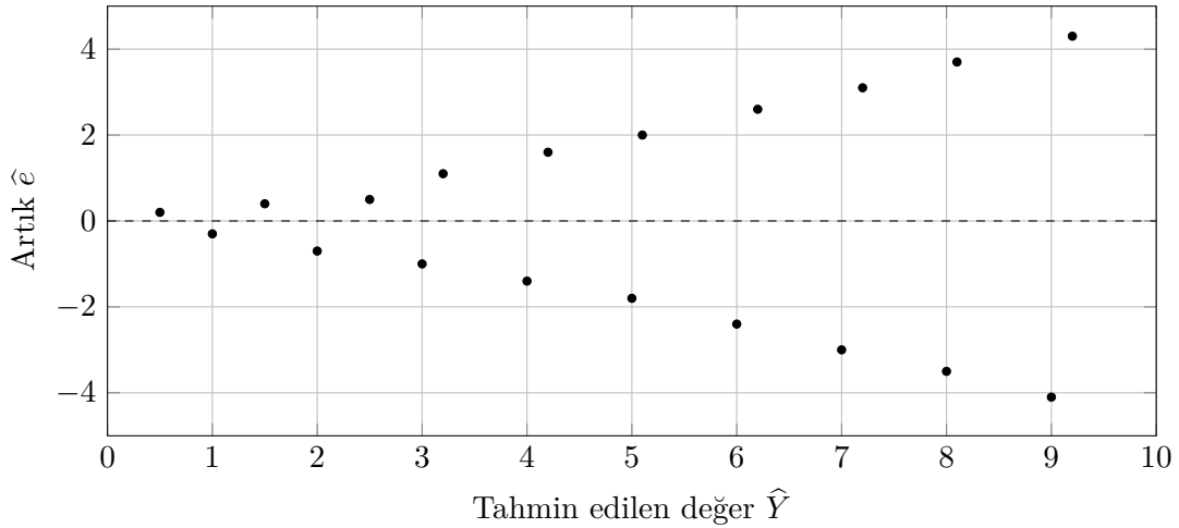
Şekil 2.4: Heteroskedastisite için tipik “açılan yelpaze” artık deseni
