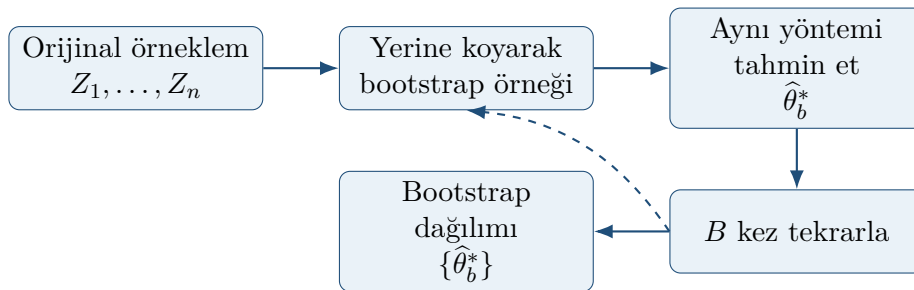
Şekil 10.1: Nonparametrik bootstrap'ın temel akışı
