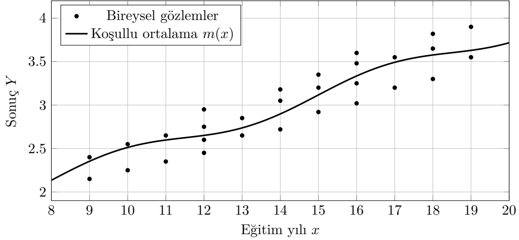
Şekil 1.2: Bireysel heterojenlik ile koşullu ortalama fonksiyonunun ayrılması
