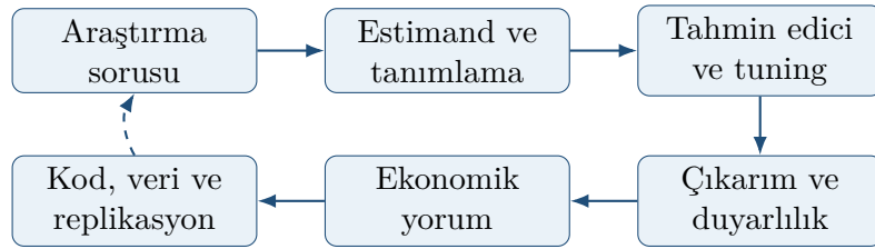
Şekil 12.5: IKT 807 boyunca kullanılan bütünleşik ampirik araştırma akışı
