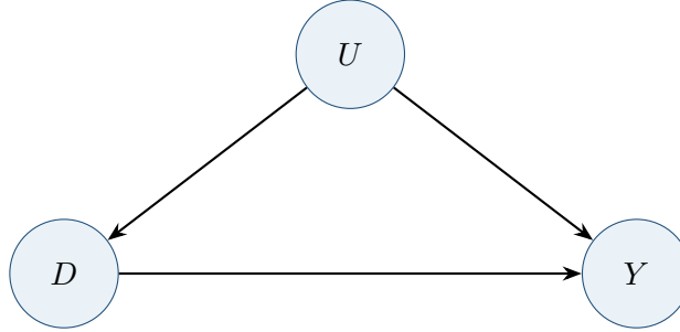
Şekil 3.2: Gözlenemeyen U hem tedaviyi hem sonucu etkilediğinde seçim/karıştırma yolu
