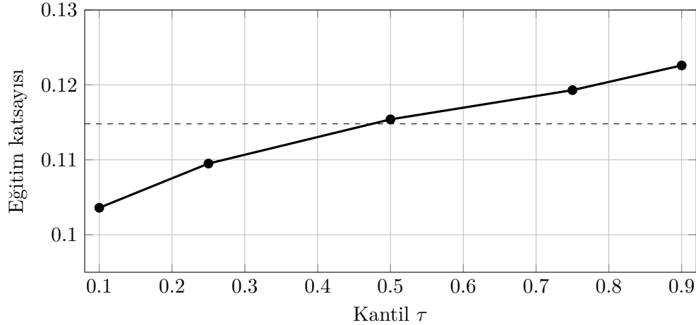
Şekil 7.4: CPS uygulamasında eğitim katsayısının kantil profili; kesikli çizgi OLS eğimini gösterir
