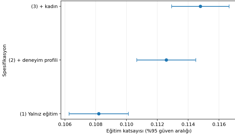
Şekil 1.8: Farklı spesifikasyonlarda eğitim katsayısı ve yüzde 95 güven aralıkları
