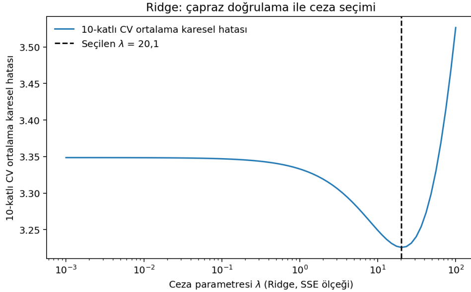
Şekil 11.2: Kontrollü örnekte Ridge ceza parametresinin 10-katlı çapraz doğrulamayla seçimi. Kesikli çizgi CV hatasının en küçük olduğu cezadır.
