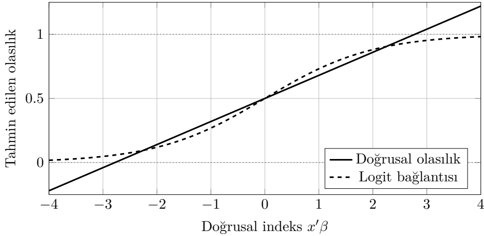
Şekil 5.1: Doğrusal olasılık modelinde sınır ihlali ve S-biçimli bağlantı fonksiyonu
