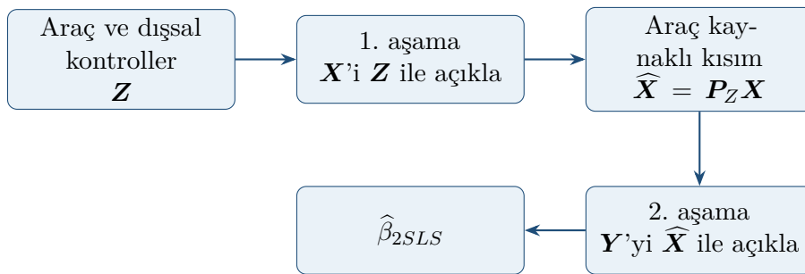
Şekil 4.2: 2SLS'nin projeksiyon mantığı
