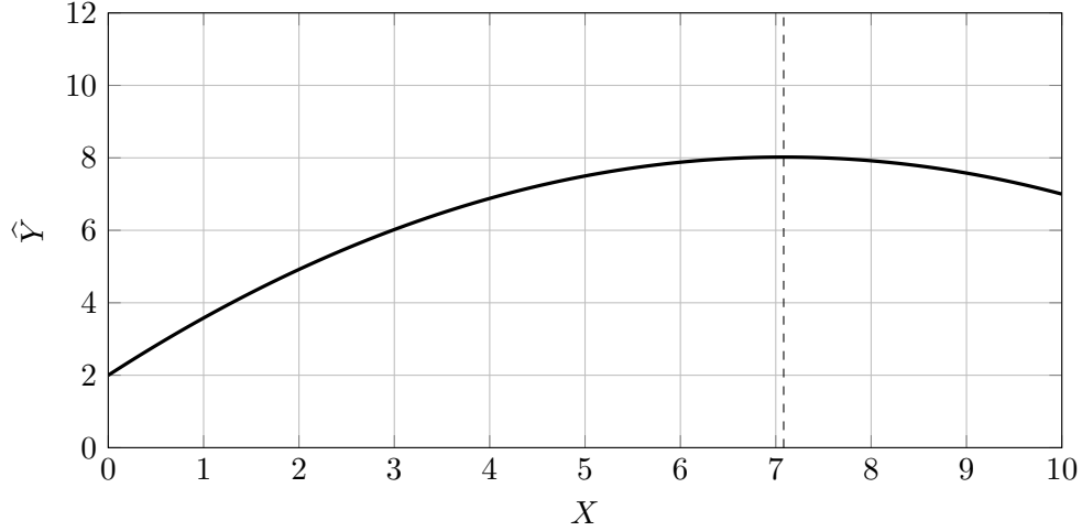
Şekil 2.2: Karesel modelde marjinal ilişkinin X düzeyine göre değişmesi
