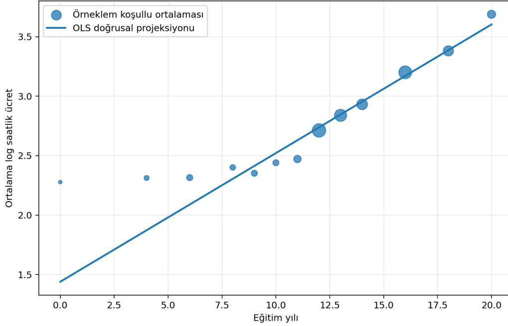
Şekil 1.7: Eğitim düzeyine göre koşullu ortalama ve OLS doğrusal projeksiyonu
