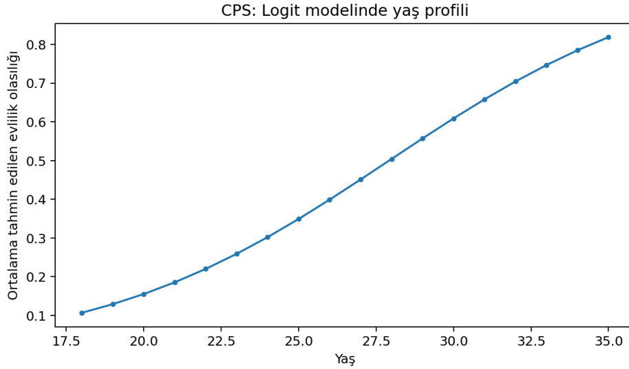
Şekil 5.4: CPS Logit modelinde yaşa göre ortalama tahmin edilen evlilik olasılığı
