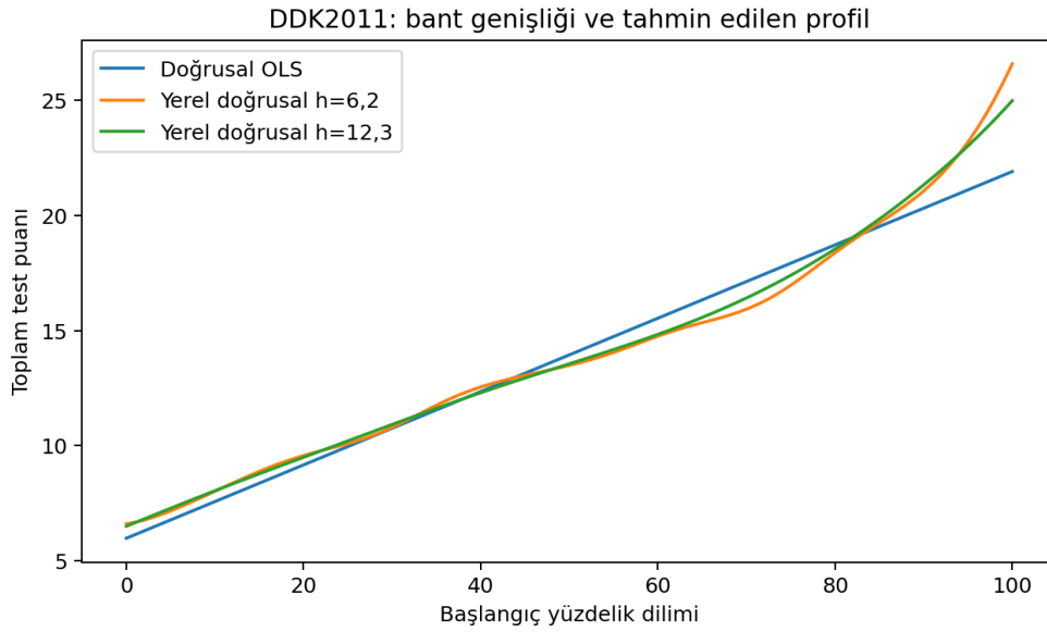
Şekil 8.4: DDK2011: doğrusal model ve iki farklı bant genişliğinde yerel doğrusal tahmin
