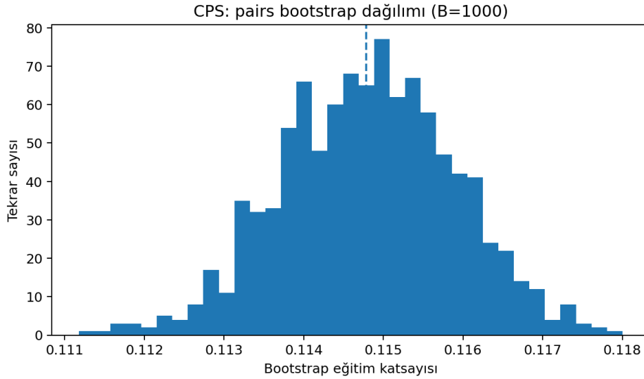
Şekil 10.3: CPS eğitim katsayısının pairs bootstrap dağılımı
