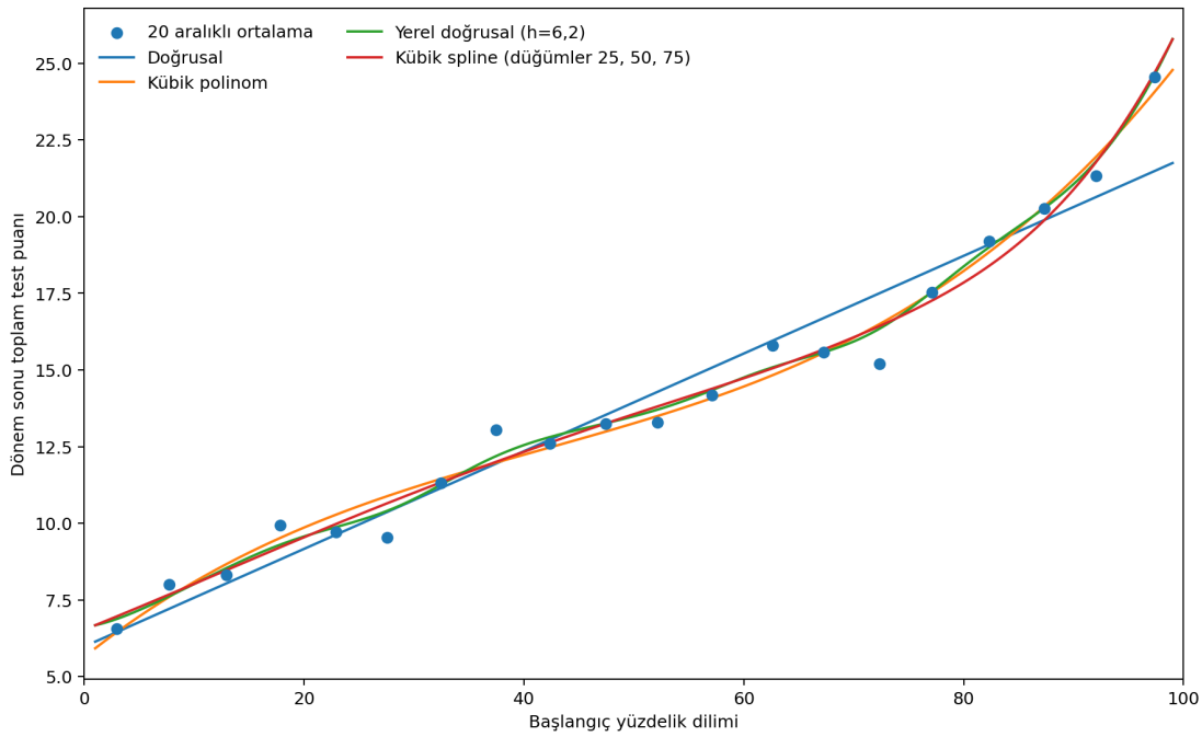
Şekil 8.3: DDK2011 verisinde doğrusal, polinom, yerel doğrusal ve spline uyumlarının karşılaştırılması
