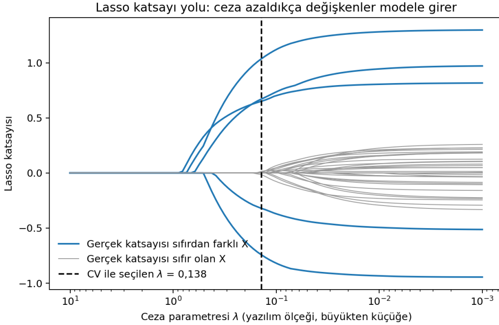
Şekil 11.1: Kontrollü örnekte (bölüm 11.14) Lasso katsayı yolu. Mavi çizgiler gerçek katsayısı sıfırdan farklı beş değişkendir; kesikli çizgi 10-katlı çapraz doğrulamayla seçilen ceza düzeyini ( \lambda_y , yazılım ölçeği) gösterir.
