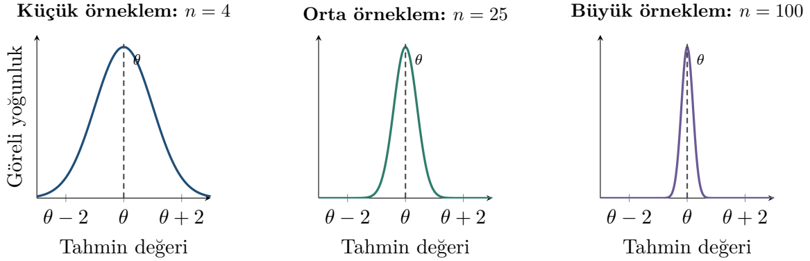
Şekil 12.12: Örneklem büyüklüğü arttıkça tahmin edicinin örnekleme dağılımının gerçek parametre çevresinde daralması. Paneller aynı merkezde çizilmiştir; farklılaşan özellik yayılımdır. Eğriler, karşılaştırmayı kolaylaştırmak için görelî yoğunluk ölçeğinde gösterilmiştir.
