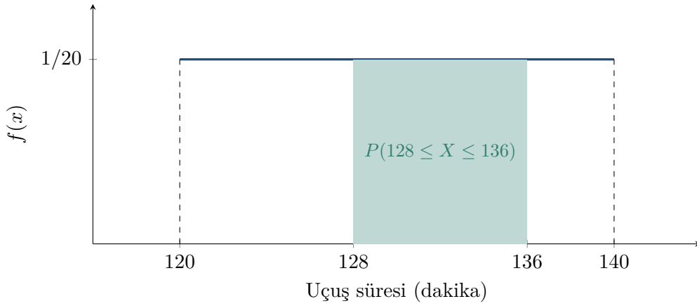
Şekil 10.4: U(120, 140) tek-düze dağılımında 128–136 dakika aralığı
