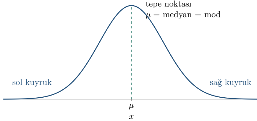
Şekil 10.6: Normal dağılımın temel çan biçimi ve simetrisi
