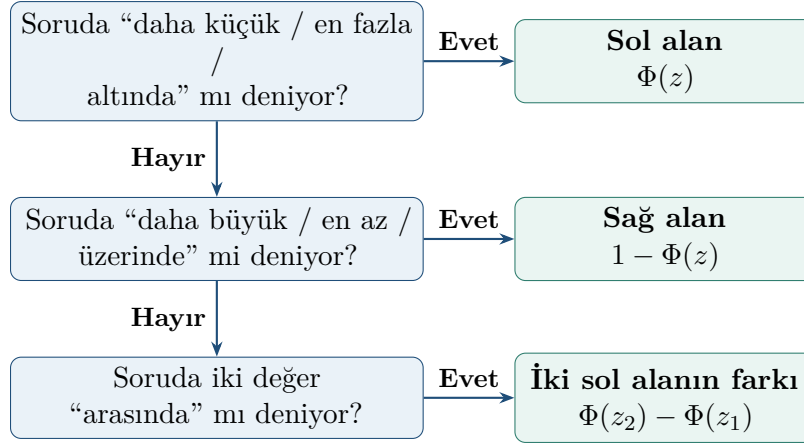
Şekil 11.6: Normal olasılık sorusunda istenen alan türünü belirleme şeması
