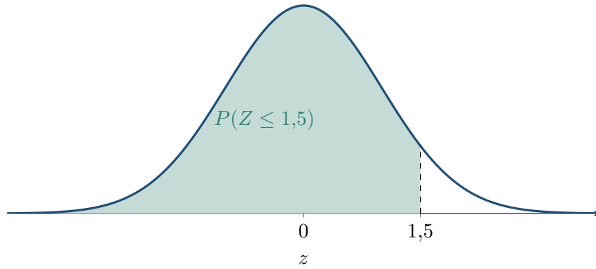
Şekil 11.2: Sol kuyruk olasılığı: istenen alan doğrudan \Phi(z) 'dir
