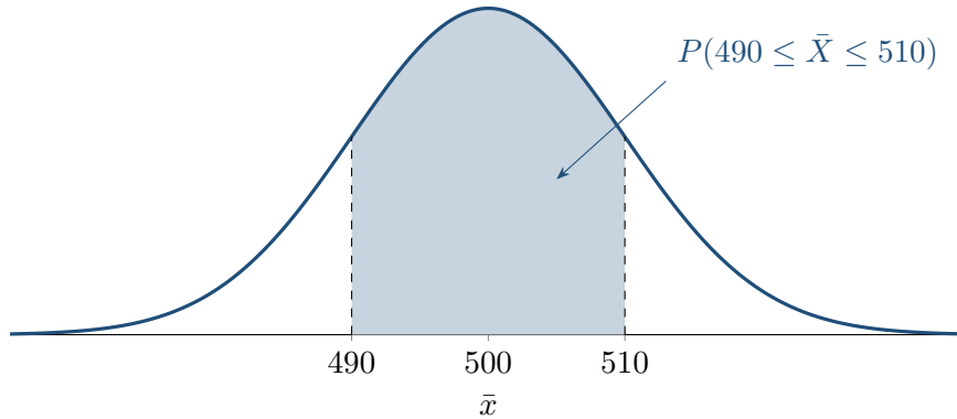
Şekil 12.9: n = 36 için örneklem ortalamasının 500 çevresindeki olasılığı
