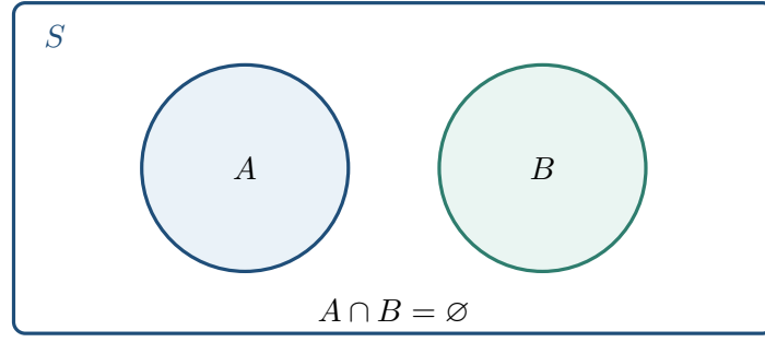
Şekil 6.11: Ortak örnek noktası bulunmayan ayrık olaylar
