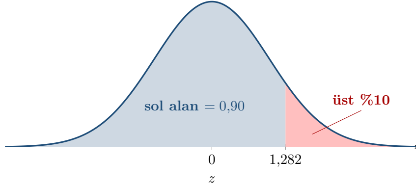
Şekil 11.5: Üst yüzdeyi ayıran eşik değerinin normal eğri üzerinde gösterimi
