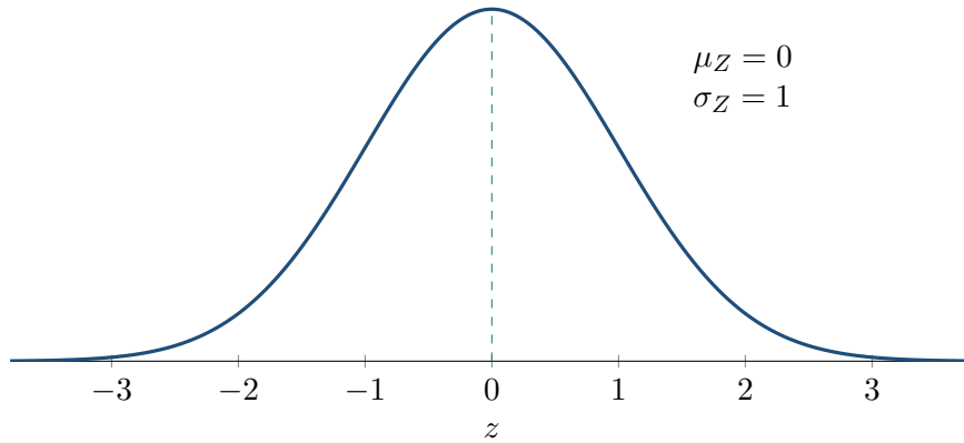
Şekil 10.10: Standart normal dağılım N(0, 1)
