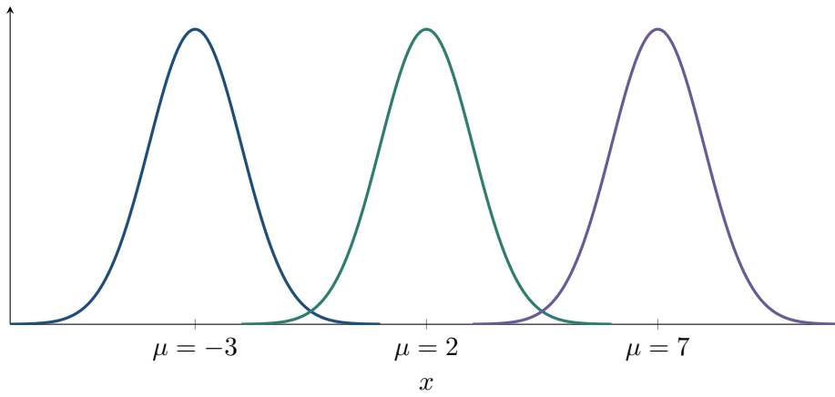
Şekil 10.7: Aynı \sigma = 1 altında farklı ortalamaların normal eğriyi yatay ekseninde taşıması
