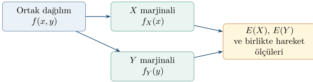
Şekil 8.12: İki değişkenli dağılımdan marjinal dağılımlara ve özet ölçülere geçiş
