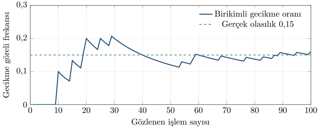
Şekil 6.6: Gecikme olasılığı 0,15 olan bir süreçte 100 işlemin birikimli gecikme oranı (tohumlu simülasyon)
