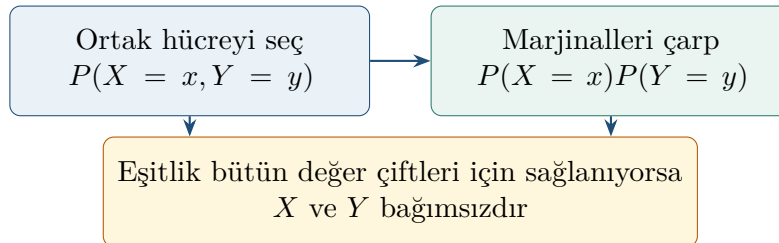
Şekil 8.13: Ortak dağılımdan rassal değişken bağımsızlığını değerlendirme mantığı
