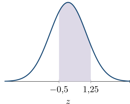
Şekil 11.3: Sağ kuyruk ve iki değer arasındaki normal olasılıkların geometrik görünümü
