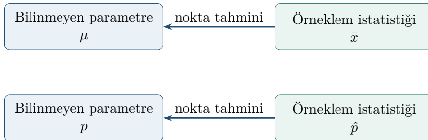
Şekil 12.4: Örneklem istatistiğinin anakütle parametresini tahmin etmesi
