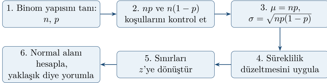
Şekil 11.9: Binomdan normal yaklaştırmaya altı adımlı çözüm şeması
