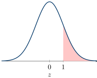
Şekil 11.3: Sağ kuyruk ve iki değer arasındaki normal olasılıkların geometrik görünümü
