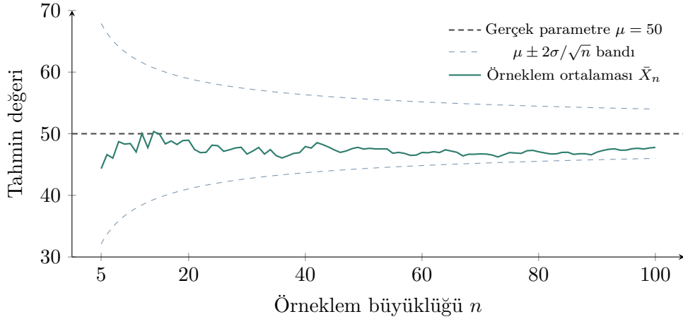
Şekil 12.13: Tutarlılığın sezgisel görünümü: tek bir örneklem büyüdükçe örneklem ortalamasının izlediği yol ve daralan \mu \pm 2\sigma/\sqrt{n} bandı ( N(50, 20^2) , tohum 217)
