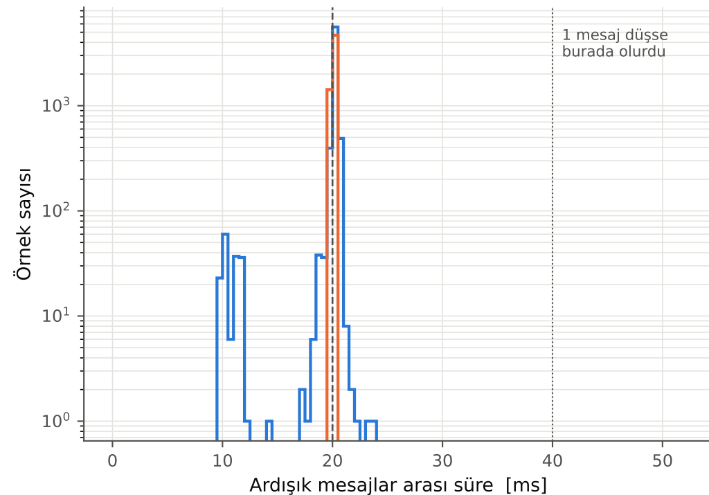
Odometri (50 Hz)
