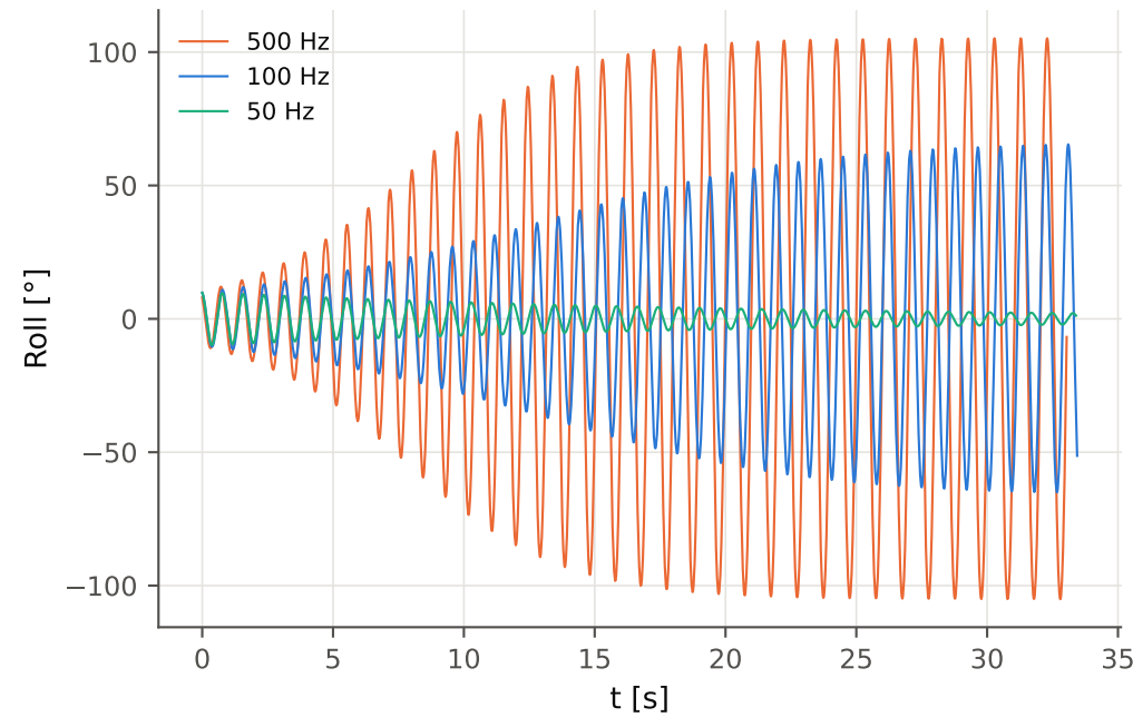
Roll, tüm kayıt (nötr, 5 m): sim hızına bağlı büyüme
