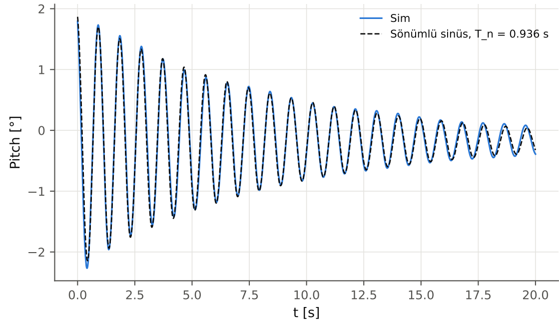
Yüzeyde pitch salınımı (başlangıç +2°)
