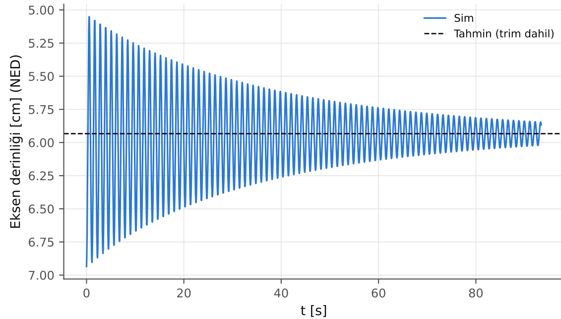
Yüzey dengesi (başlangıç: denge + 1 cm)
