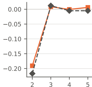
SiH 4 , IP 2 (sCI 18.17 eV)
