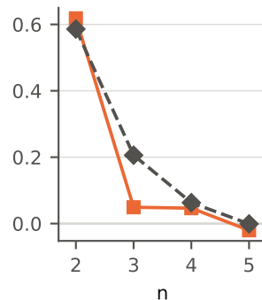
SiH 4 , IP 2 (sCI 18.17 eV)
