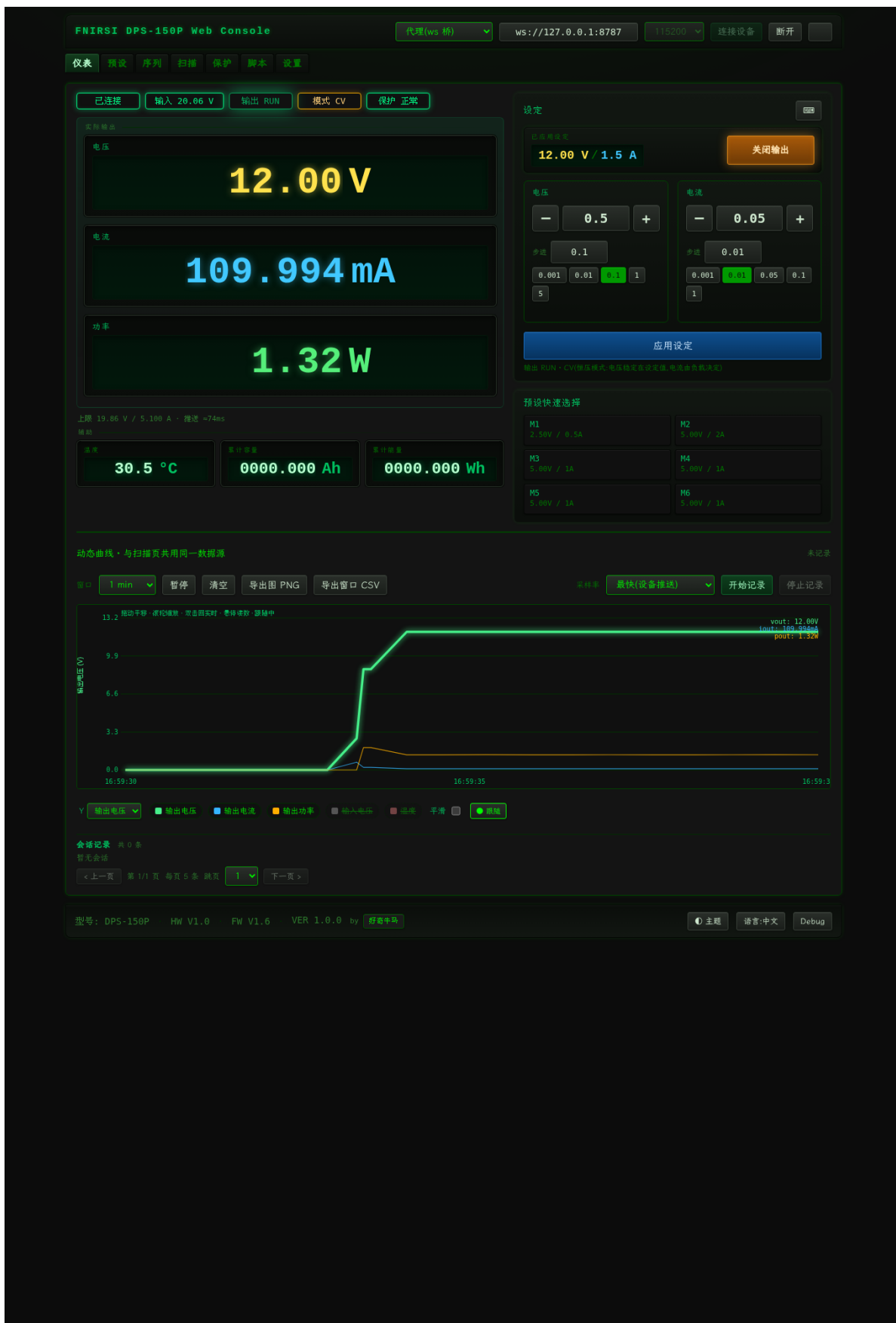
Figure 1: 仪表页 (暗色, 真机数据)
