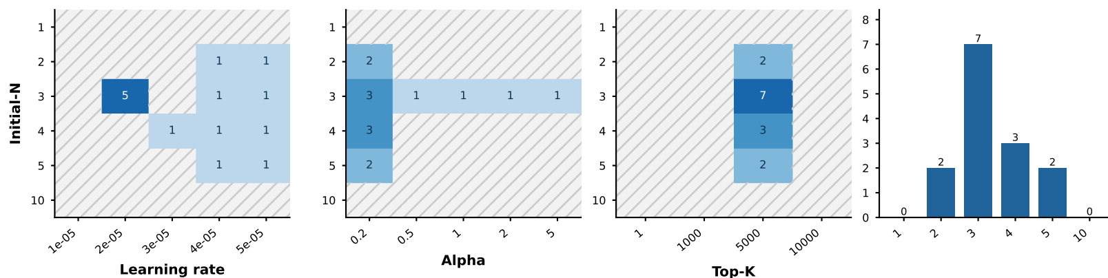
Initial-N
