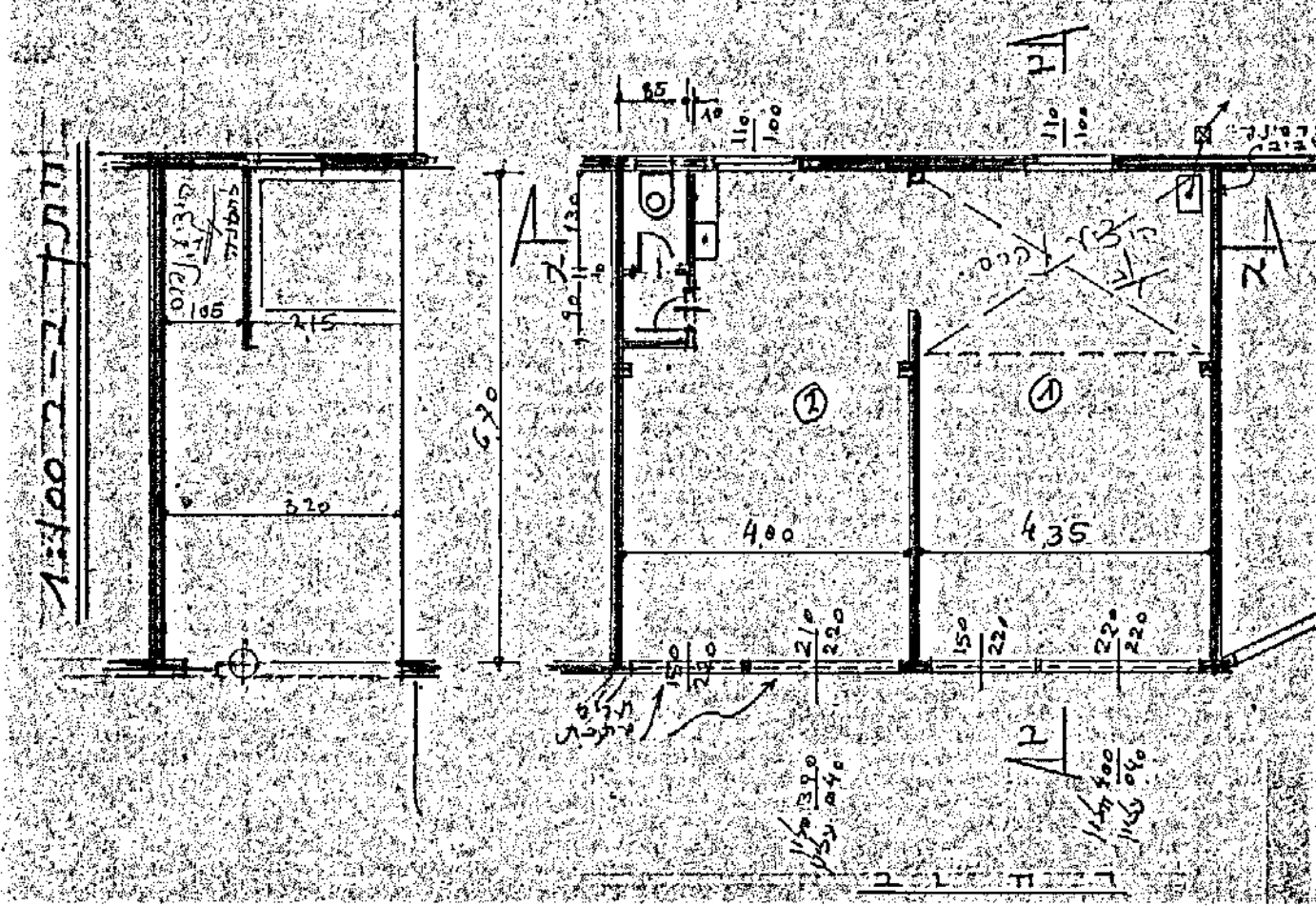
תכנית 1:100
