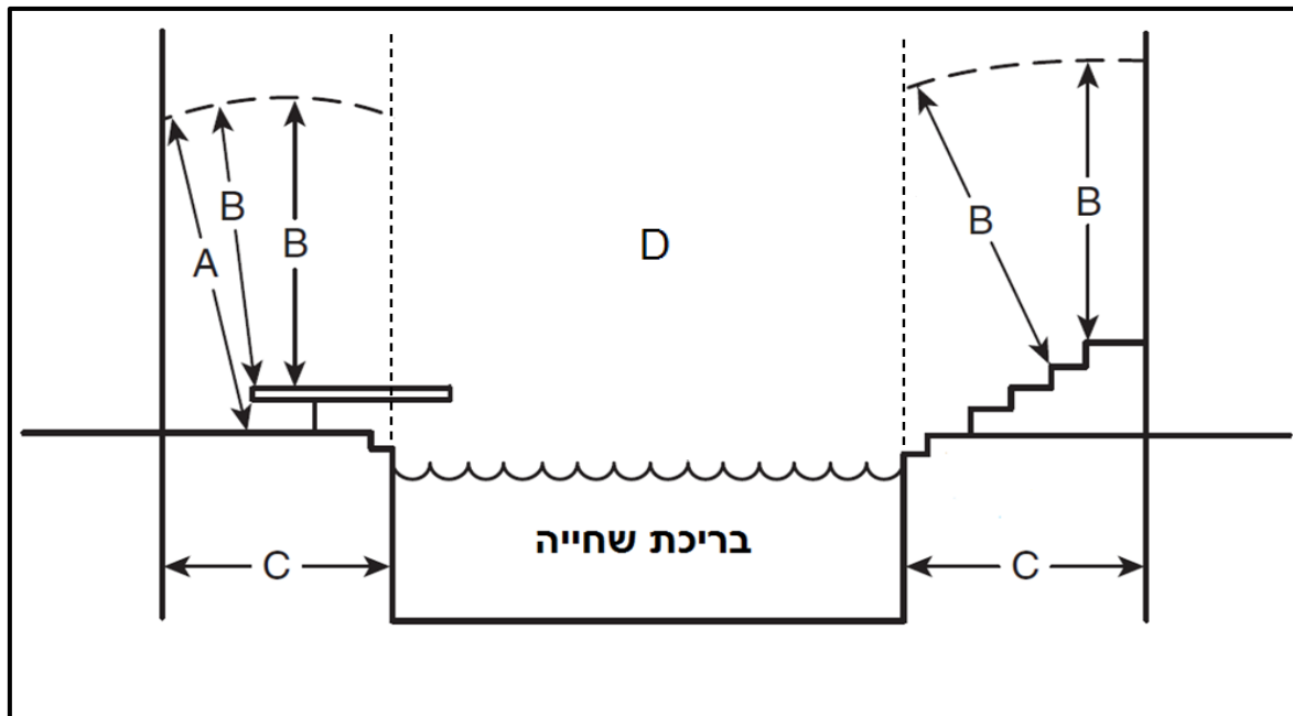
איור 1: בניית בריכת שחייה בקרבת רשת החשמל.
