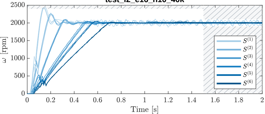
test_l2_e16_h10_40k
