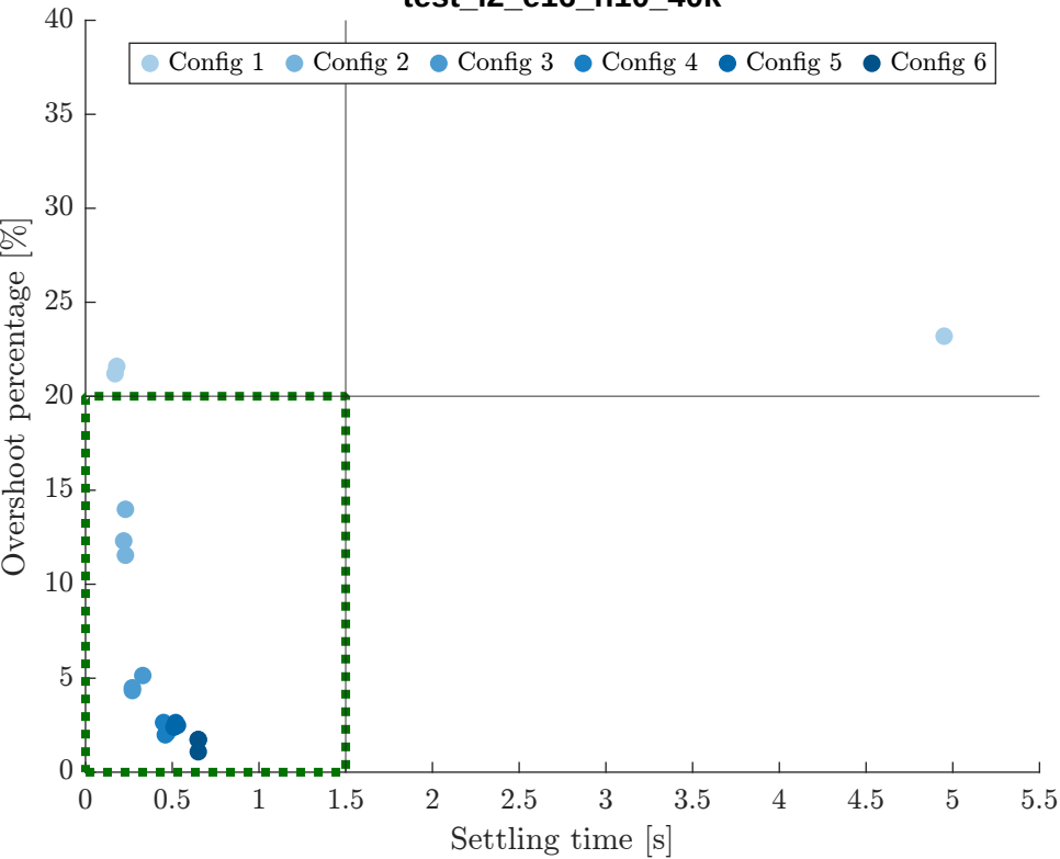
test_l2_e16_h10_40k
