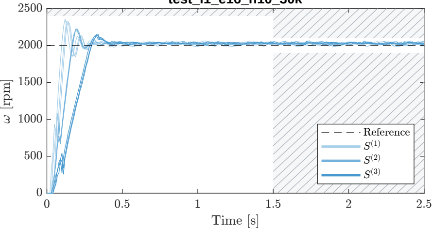
test_l1_e16_h10_30k
