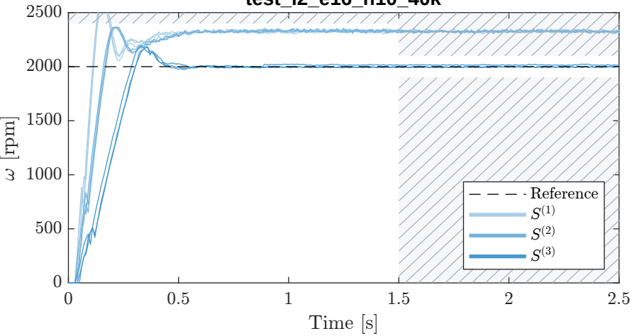
test_l2_e16_h10_40k
