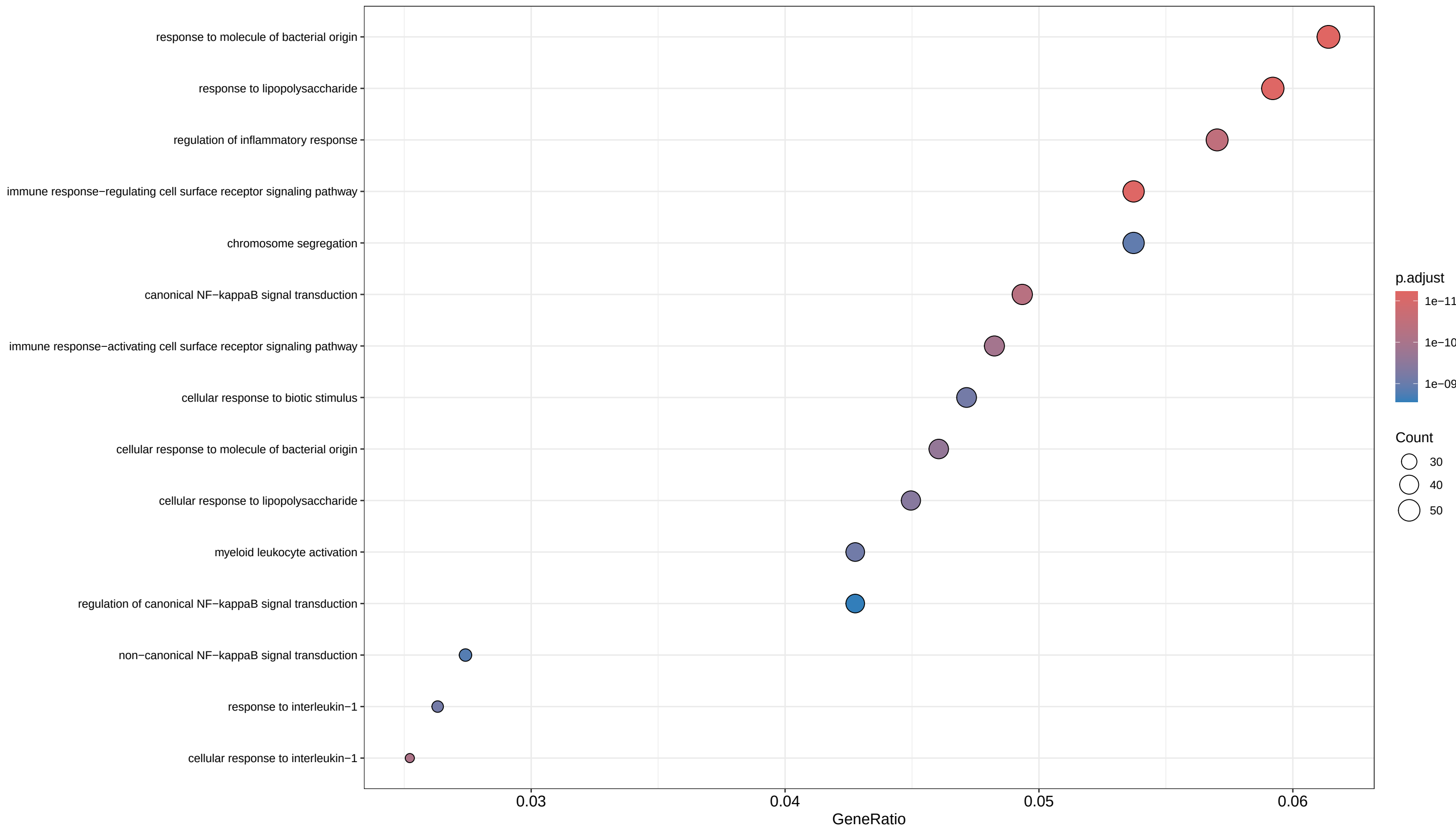
GSE207177_.... GO BP Up
