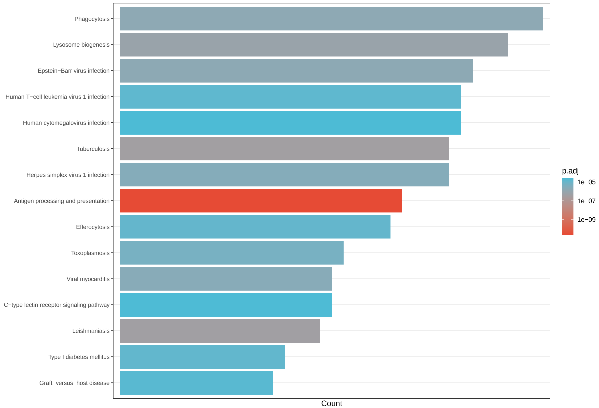
GSE207363_.... KEGG (bar)
