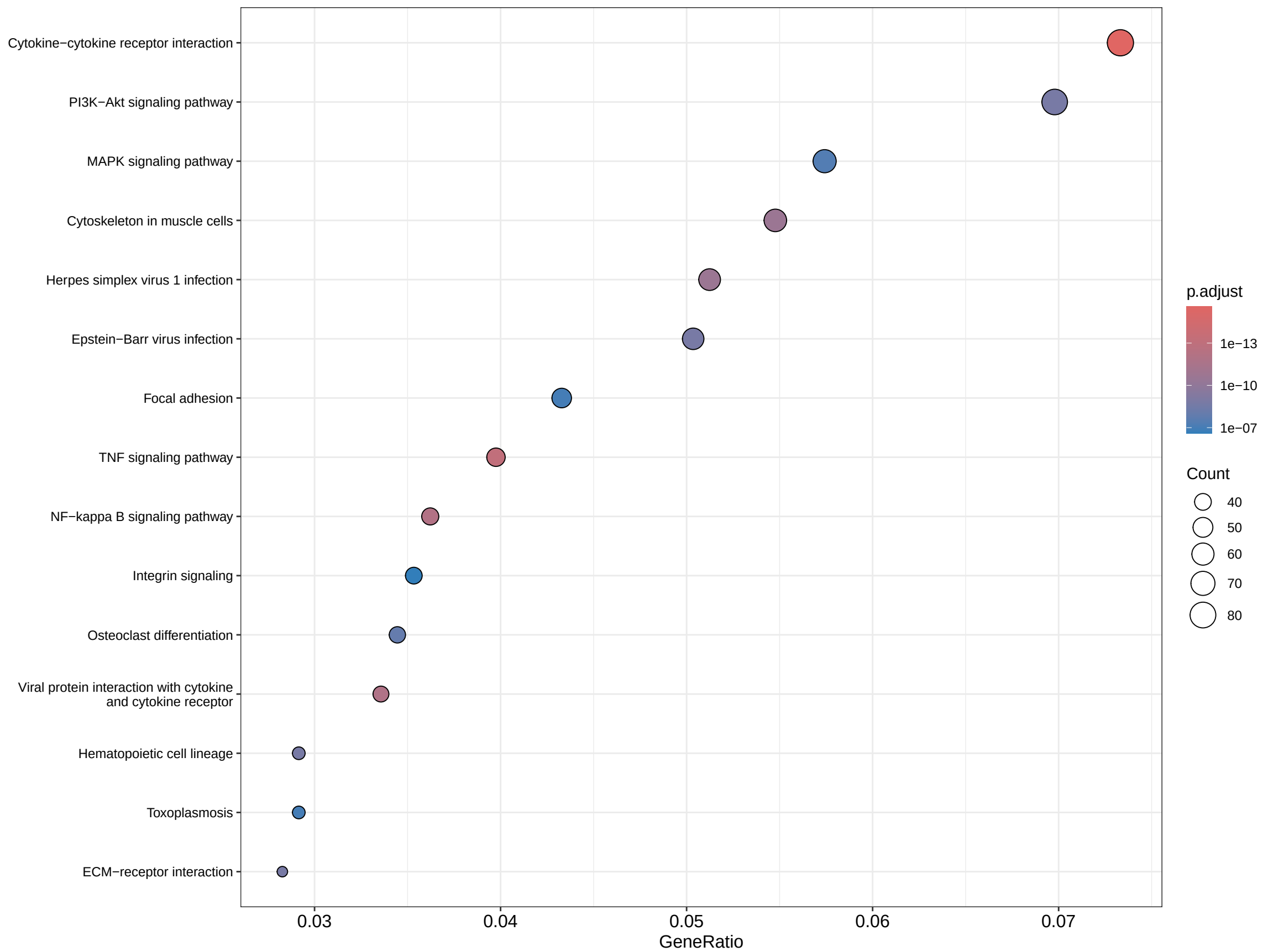
GSE267388 KEGG
