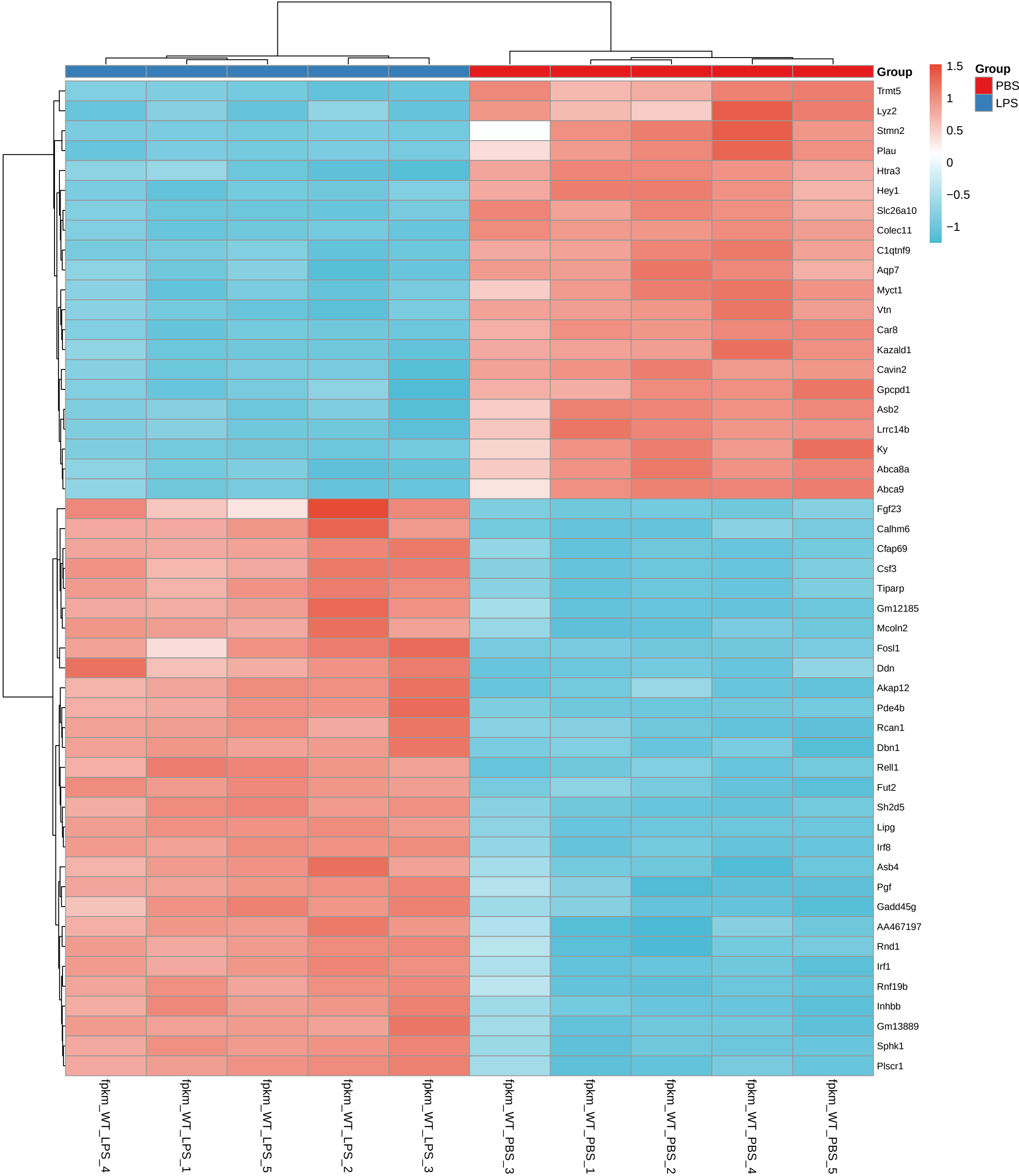
GSE267388 Top 50 DEGs
