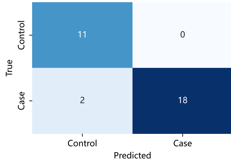
MLP (PyTorch)
