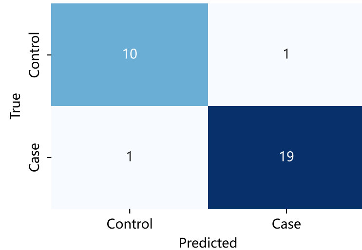
LASSO
