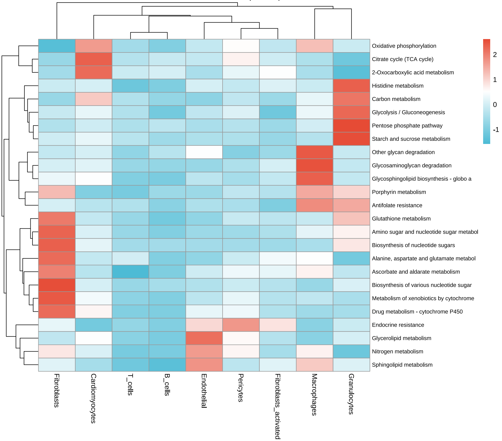
GSE207177 细胞类型代谢活性(AUC Cell )
