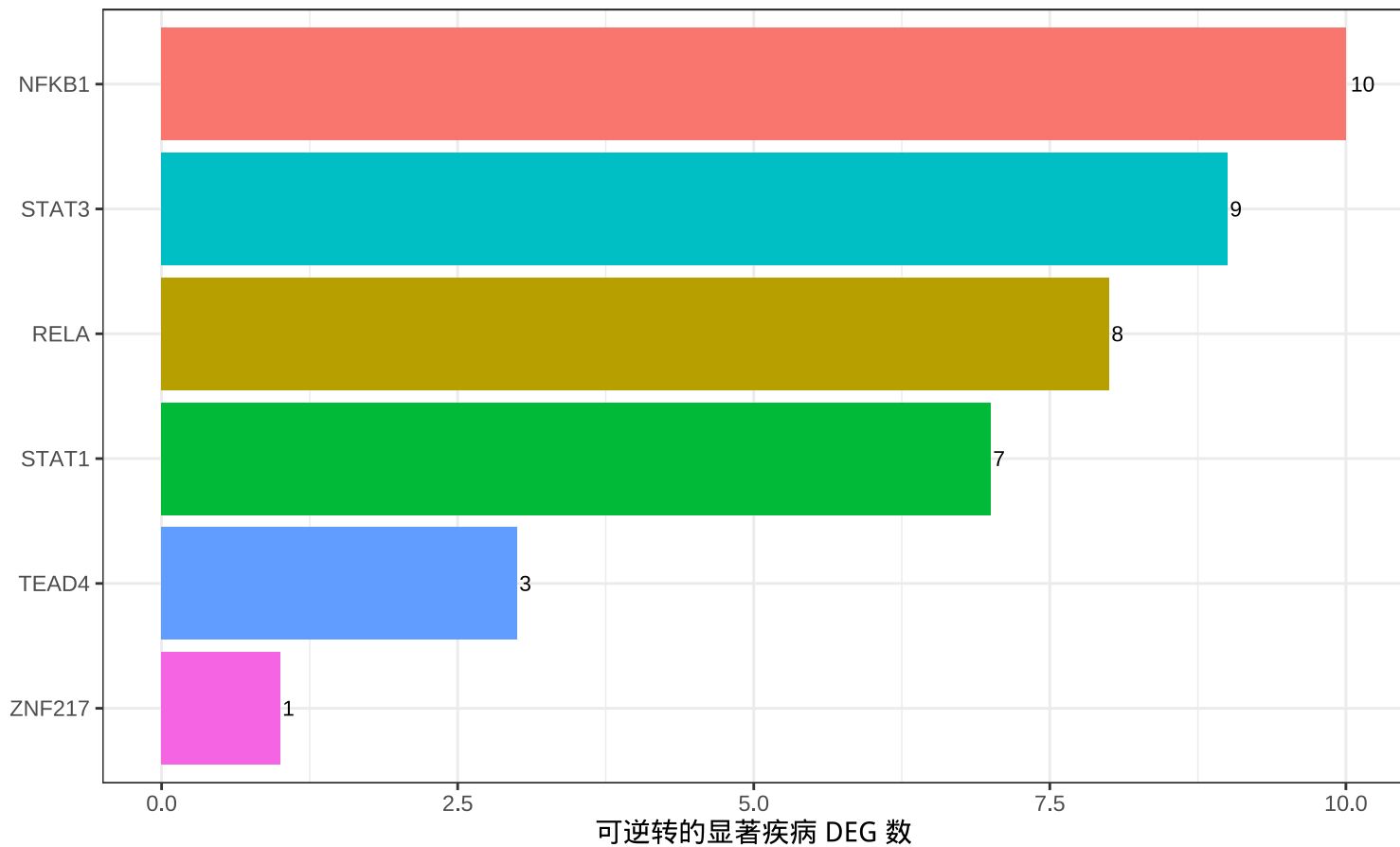
GSE79962 虚拟敲除：各 master TF 可逆转的显著疾病基因数
