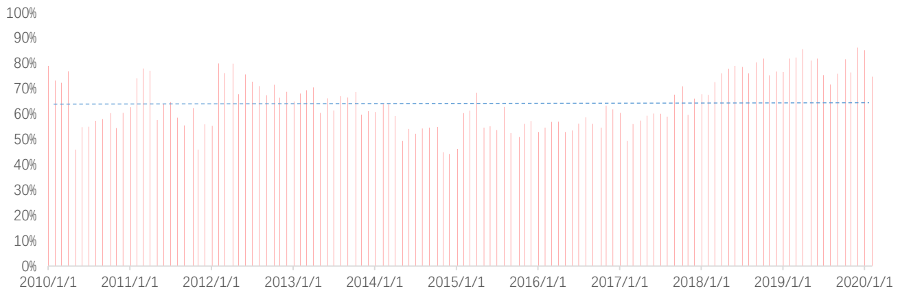
图 26：策略持仓的长期动量因子暴露水平
