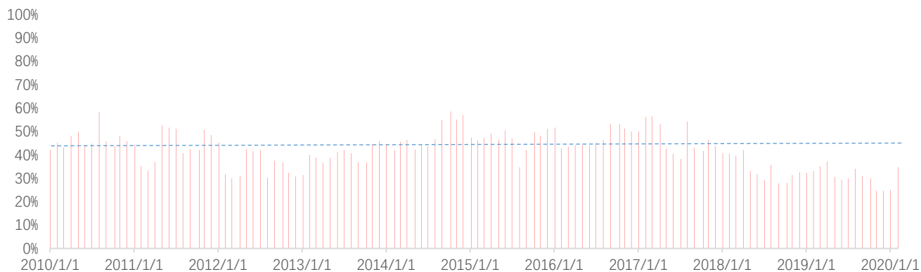
图 25：策略持仓的 BP 因子暴露水平
