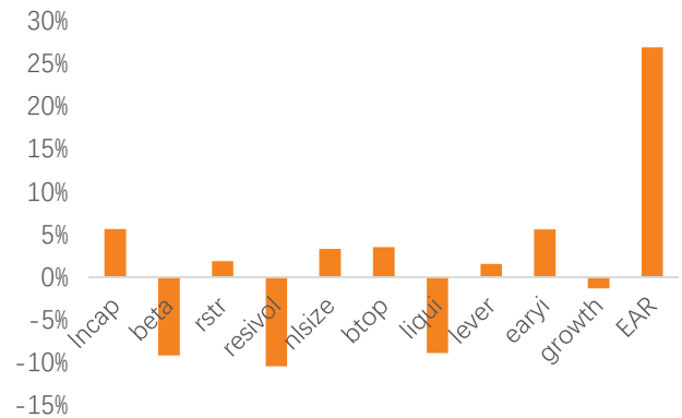
图 9：JOR 因子与 Barra 风格因子秩相关系数
