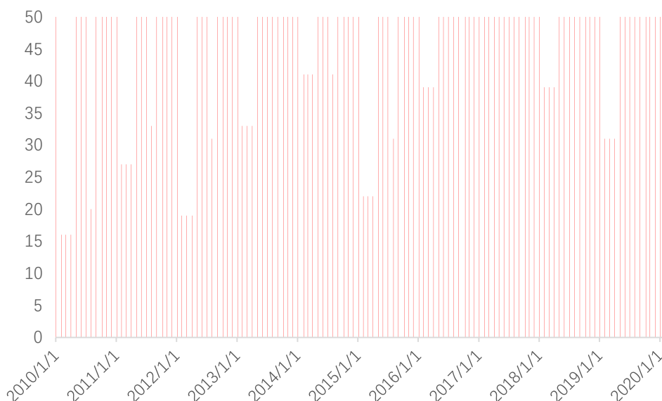
图 22：持仓上限为 50 只约束下每期的实际入选股票数量
