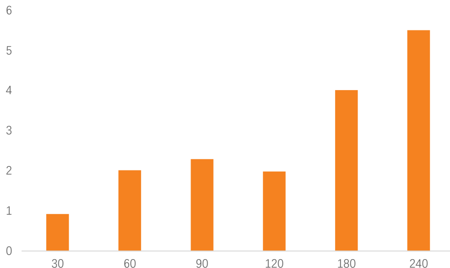
图 3：美股市场在不同持有期下的 EAR spread
