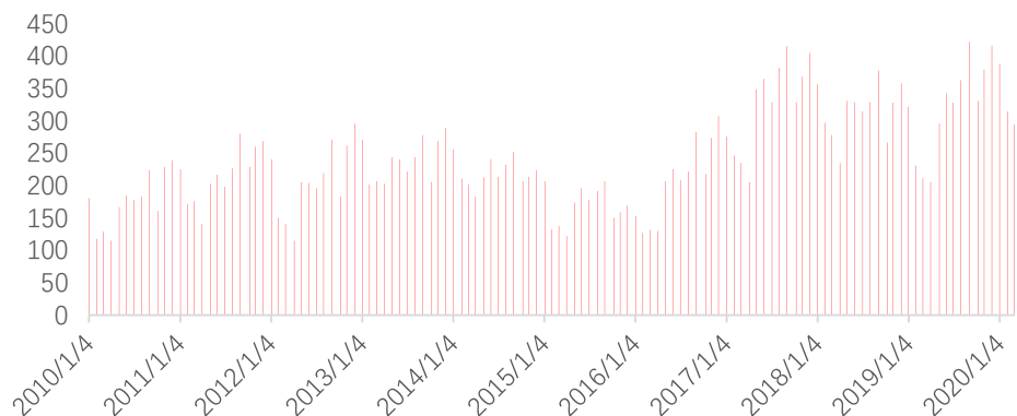
图 16：超预期样本空间样本数的时序分布
