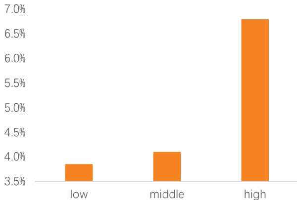
图 15：不同断层因子分组下财报超预期事件的超额收益水平
