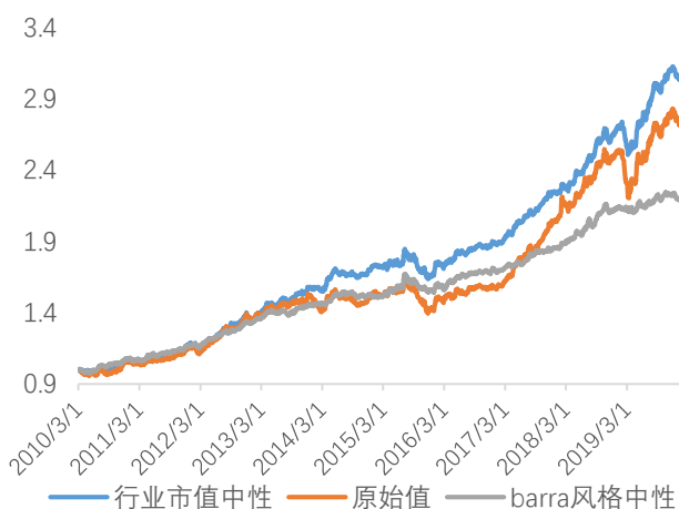
图 6：JOR 因子在不同中性化要求下的多空对冲净值（分 10 组）
