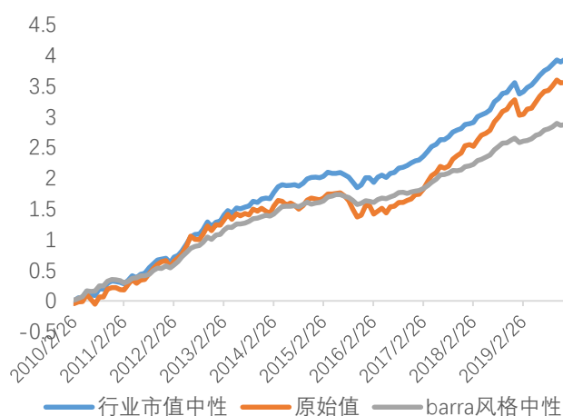
图 7：JOR 因子在不同中性化要求下的 IC 累计图
