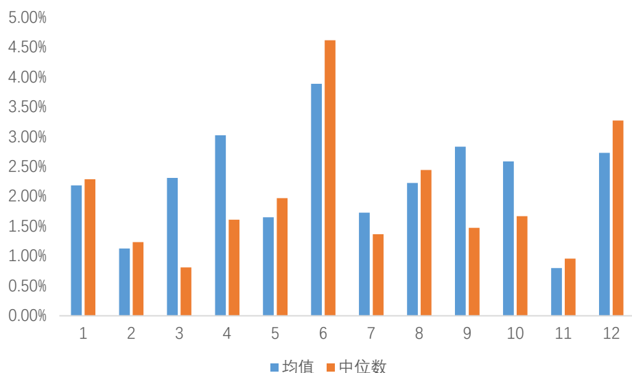
图 20：净利润断层金股组合分月相对中证 500 收益的中位数及均值
