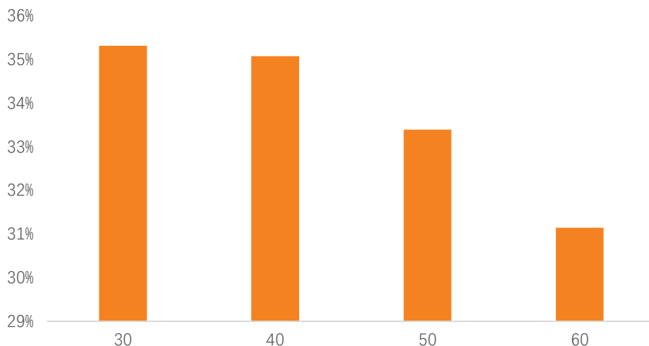
图 21：不同持仓上限约束下的组合年化收益
