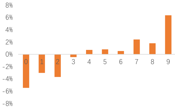
图 8：行业市值中性化后 JOR 因子十组分档年化超额收益
