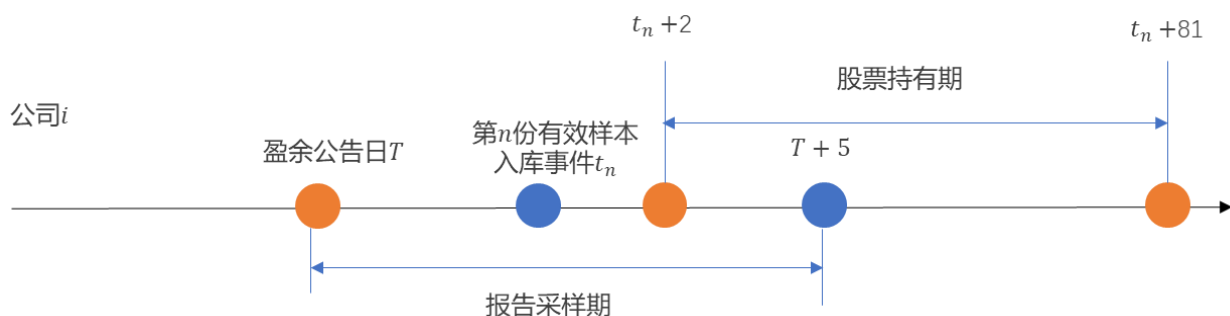
图 14：超预期事件触发流程
