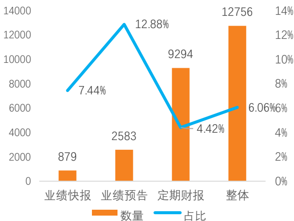
图 12：超预期分析师样本不同类型报告下的数量和占比分布
