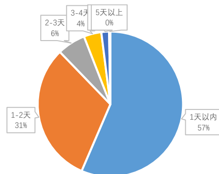
图 11：有效点评报告撰写时间与入库时间时滞差统计
