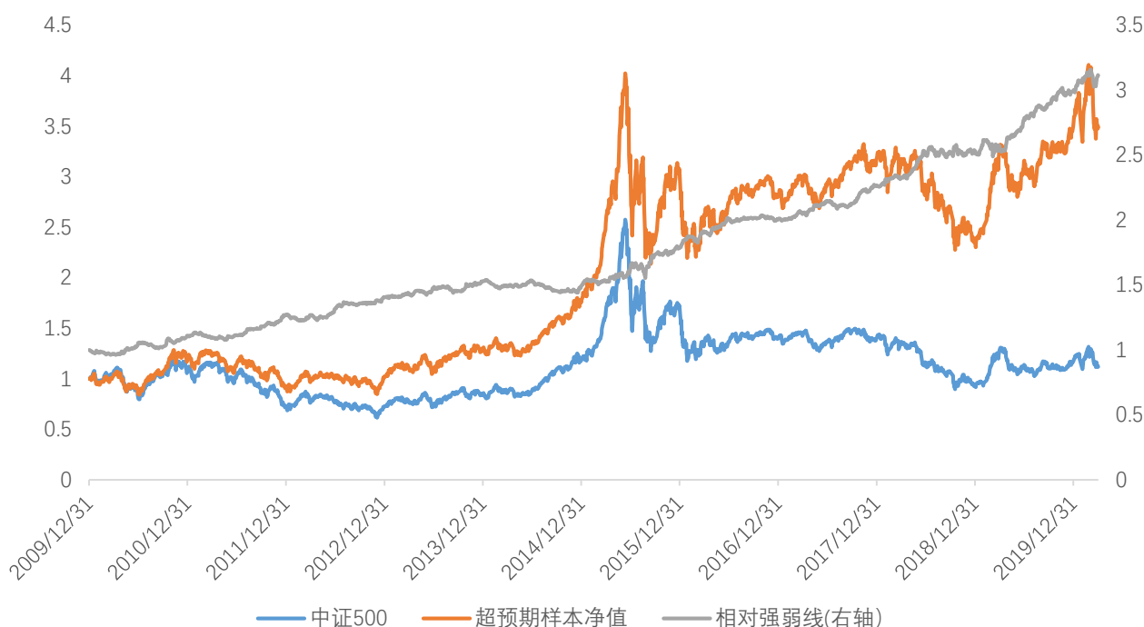
图 17：超预期样本空间相对中证 500 指数的表现
