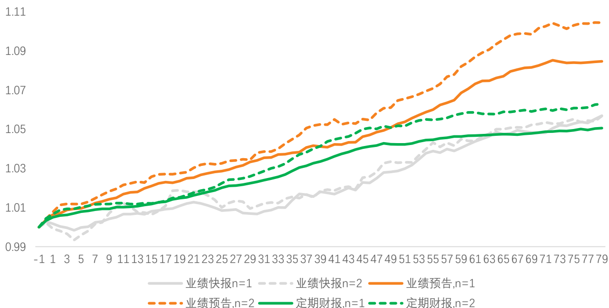
图 15：不同 n 取值下不同类型超预期事件的超额收益表现
