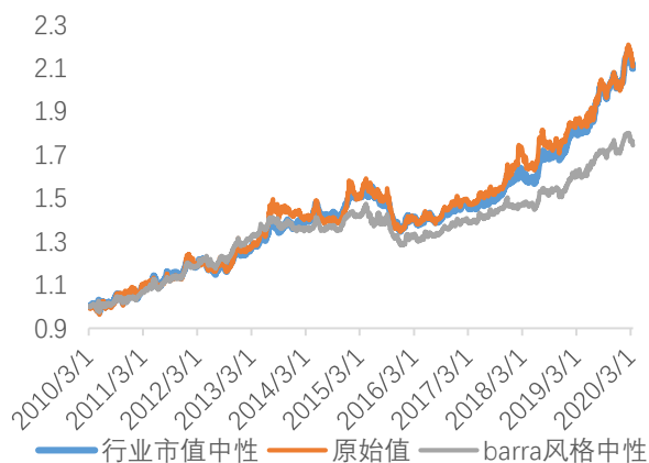
图 4：EAR 因子在不同中性化要求下的多空对冲净值（分 10 组）
