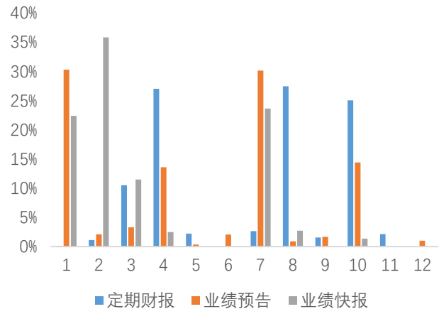
图 13：超预期分析师样本不同类型报告在不同月份的分布情况
