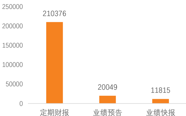
图 10：不同类型的有效点评报告的分布统计
