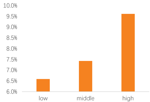
图 16：不同断层因子分组下预告超预期事件的超额收益水平
