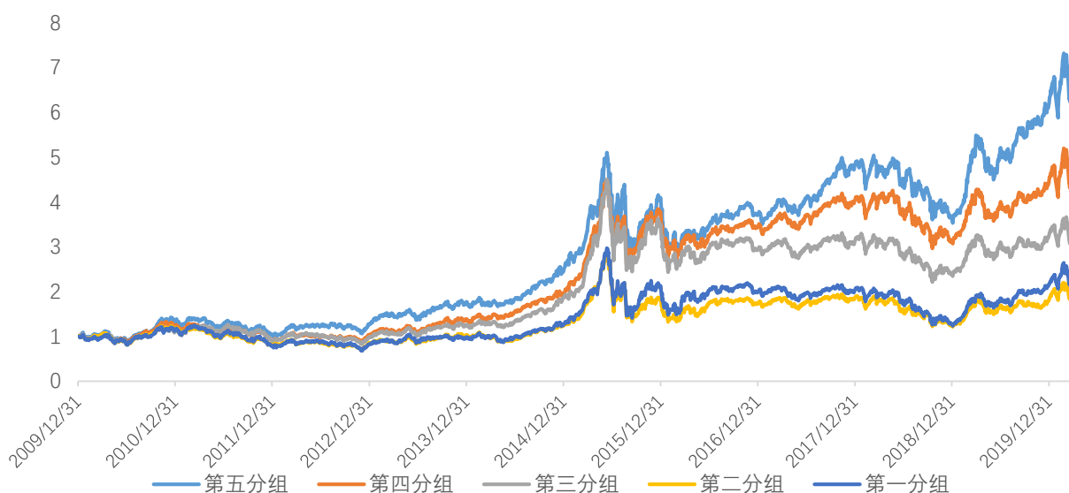
图 18：超预期样本空间在 JOR 不同分组下的业绩表现
