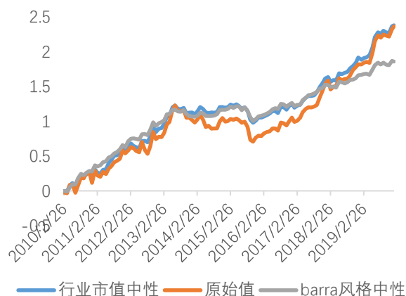
图 5：EAR 因子在不同中性化要求下的 IC 累计图
