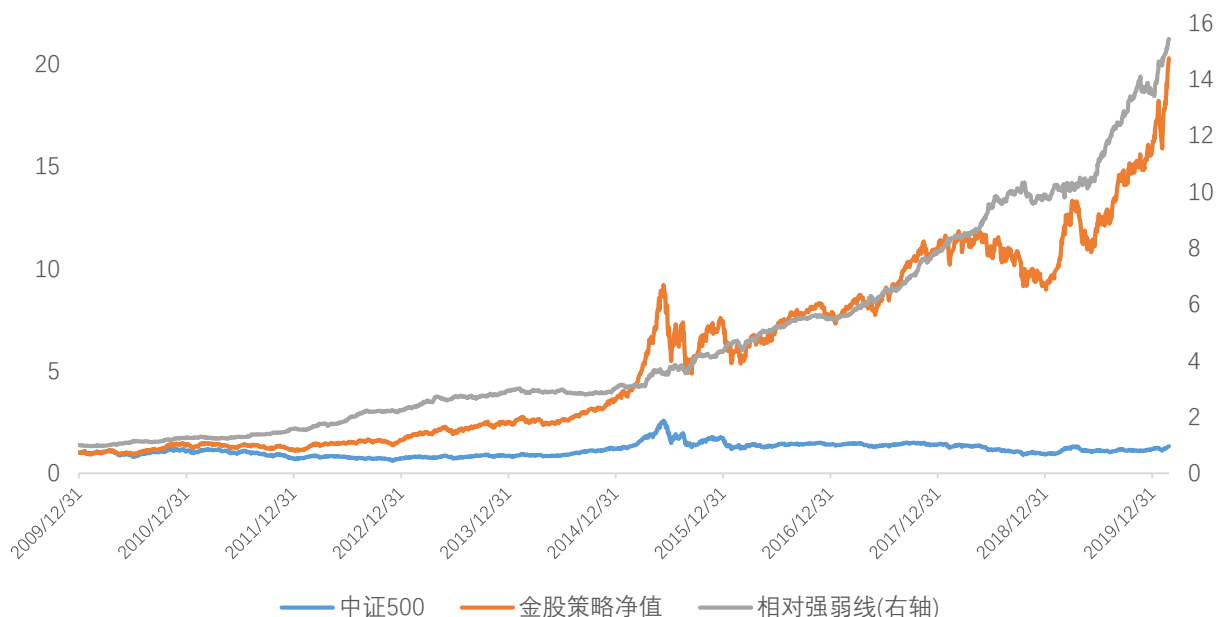
图 19：净利润断层金股策略相对中证 500 业绩表现
