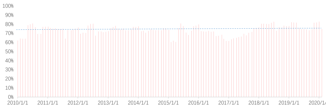
图 24：策略持仓的市值因子暴露水平
