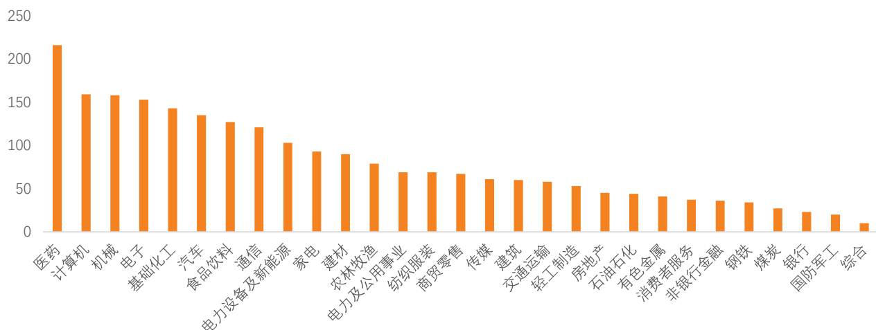
图 23：净利润断层选股组合行业入选次数分布
