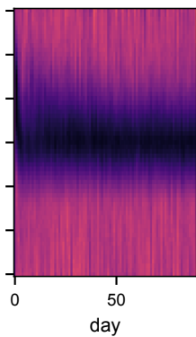
CG
