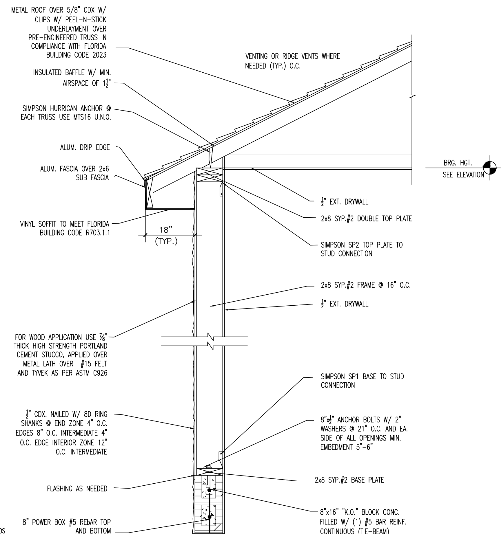
ENTRY DETAIL SCALE: N.T.S.
