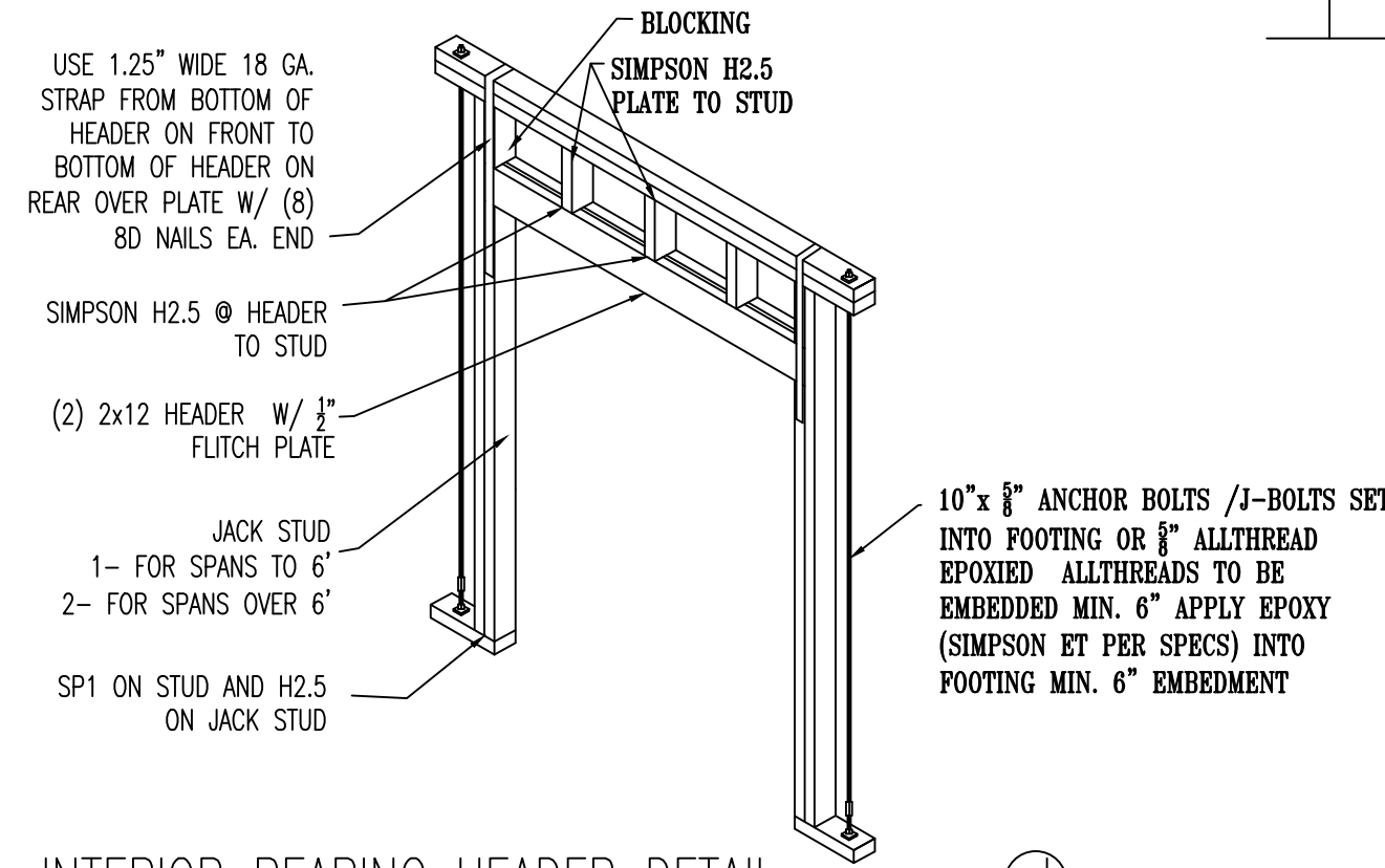
INTERIOR BEARING HEADER DETAIL SCALE: N.T.S.
