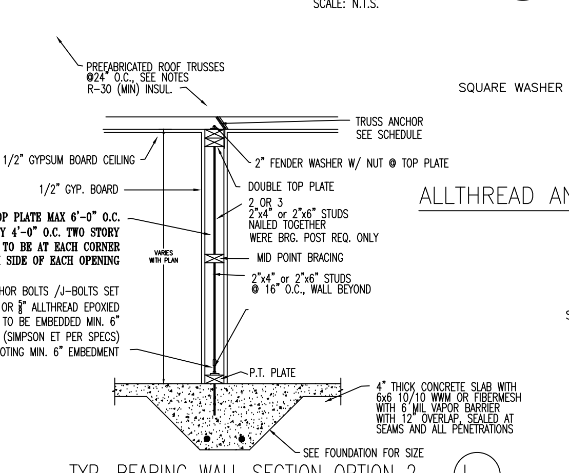
TYP. BEARING WALL SECTION OPTION 2 SCALE: N.T.S.
