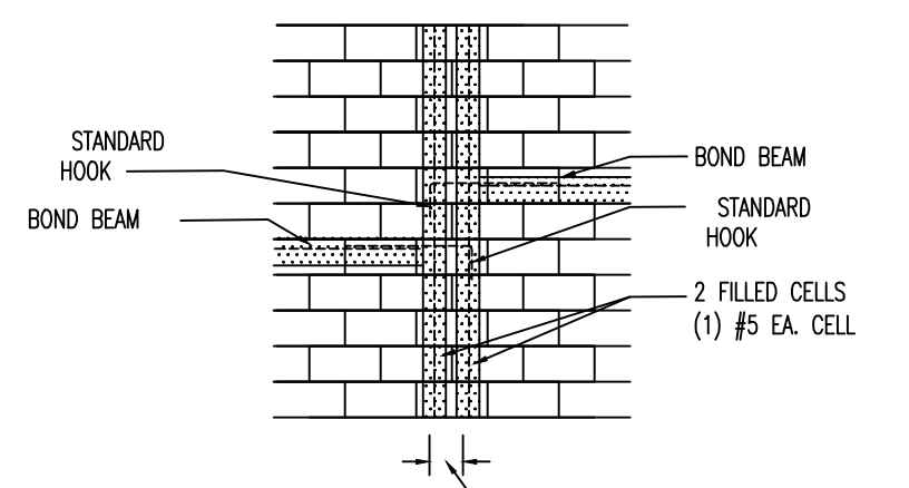
CHANGES IN BOND BEAM HGT. N.T.S.
