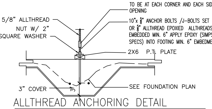
ALLTHREAD ANCHORING DETAIL SCALE: N.T.S.
