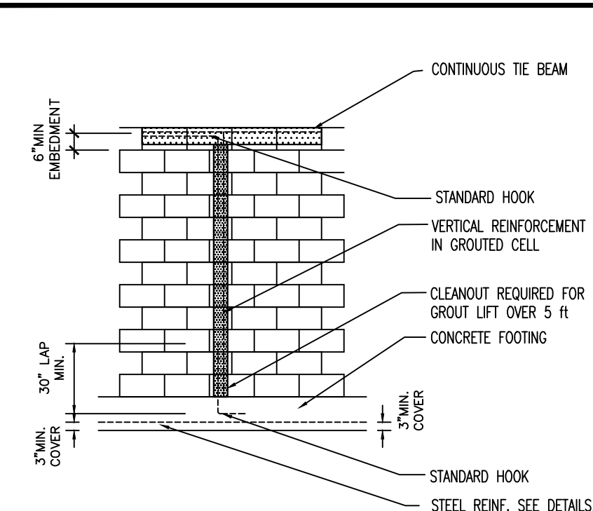
POURED CELL DETAIL N.T.S.
