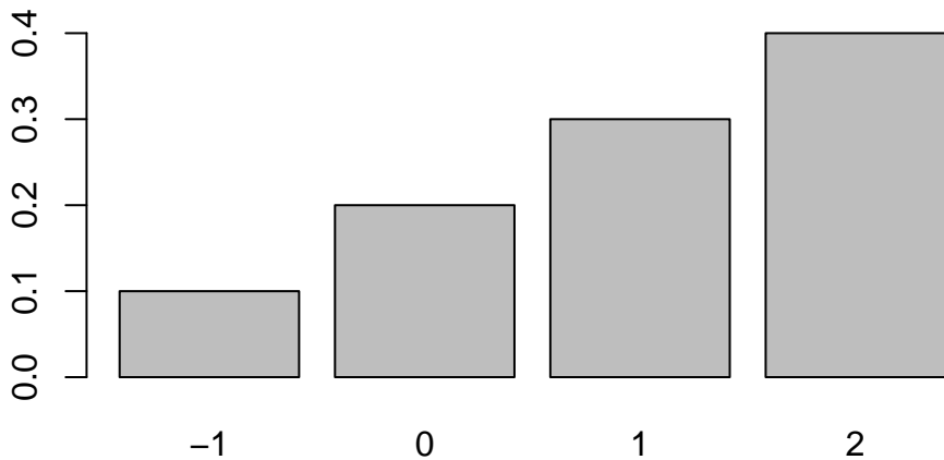
pmf of Y
