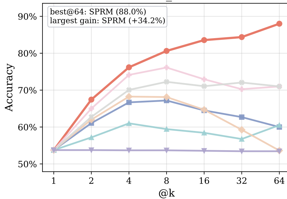
mmlu_stem
