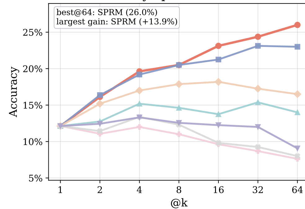
olympiadbench
