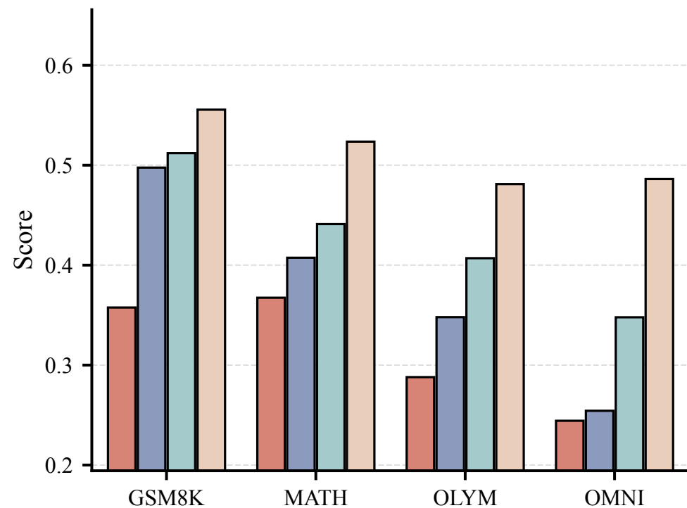
Error Acc
