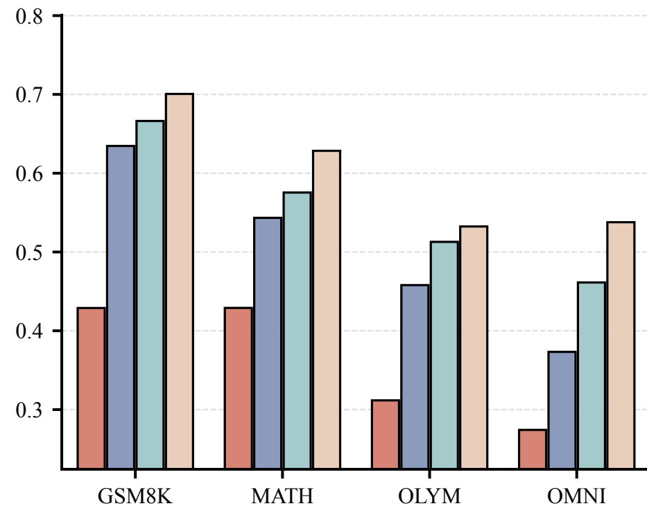
F1 Score
