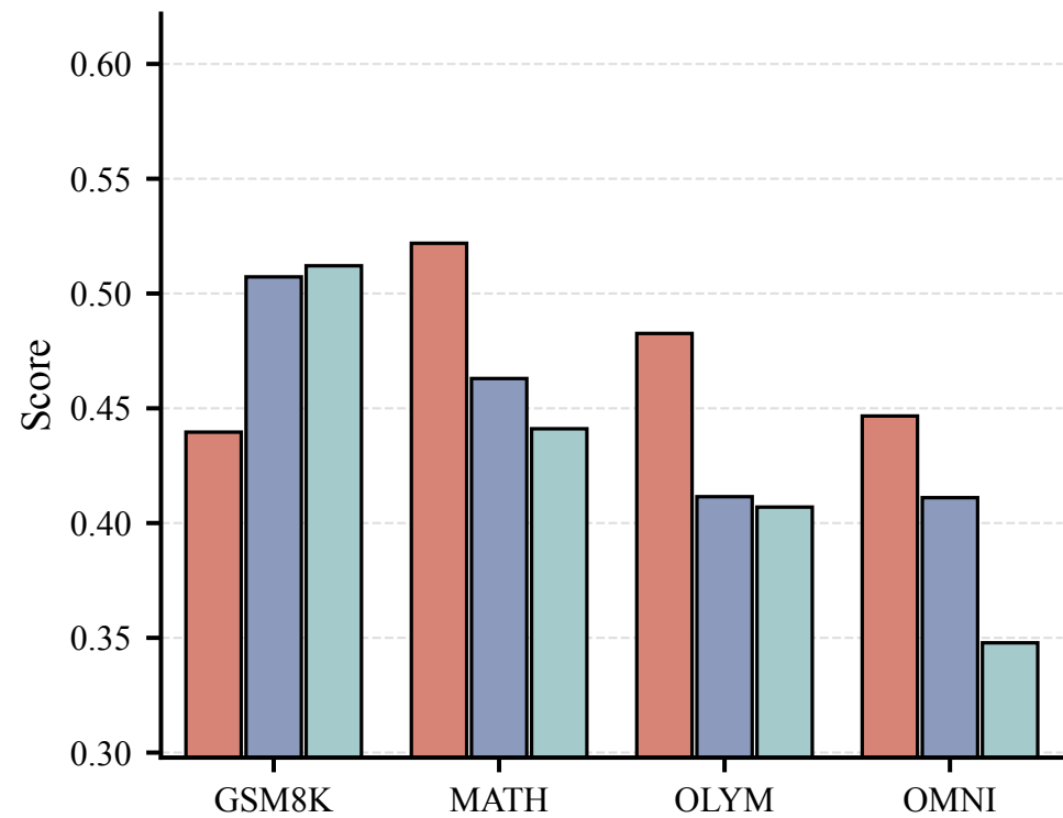
Error Acc
