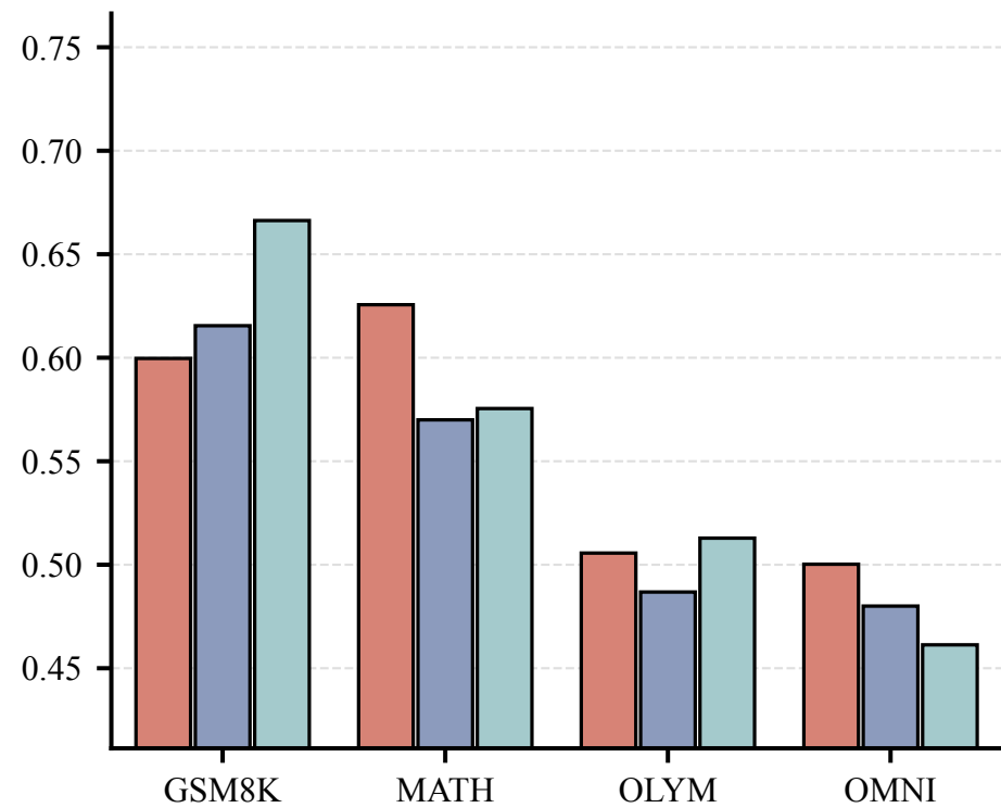
F1 Score
